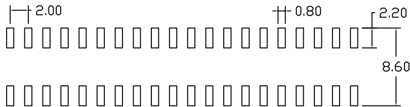
P.C.B LAYOUT
