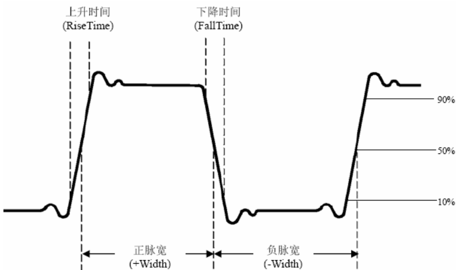
图 5-56: 时间参数定义示意
