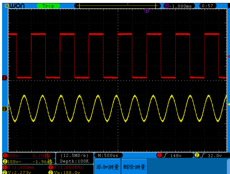
图6-1：自动测量波形
