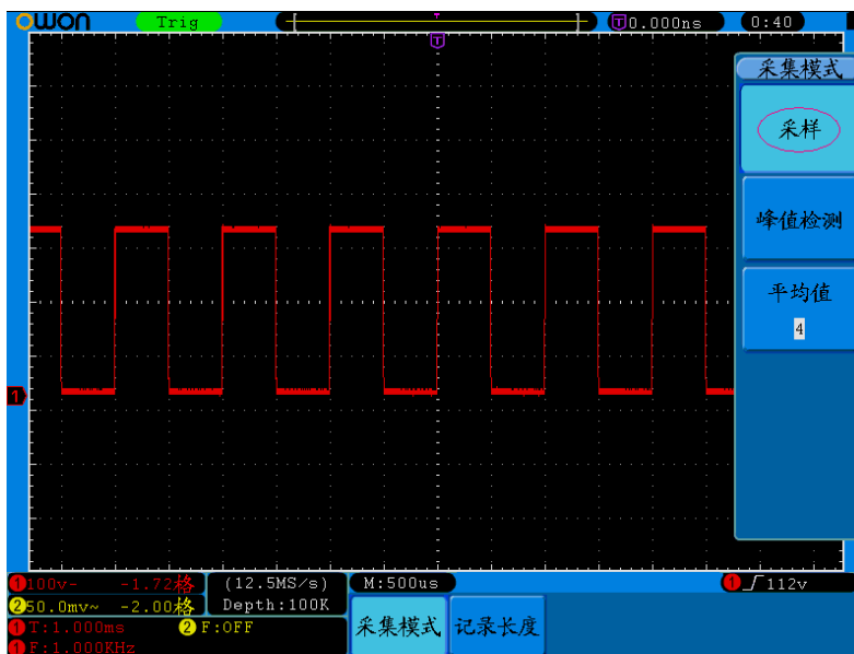
图 5-27: 普通采样方式显示，检测不到毛刺。
