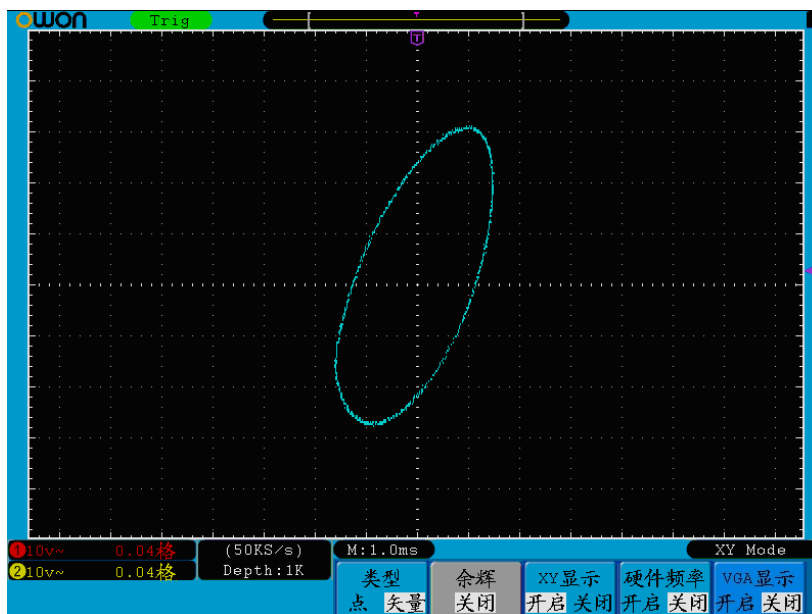
图5-33: XY显示模式
