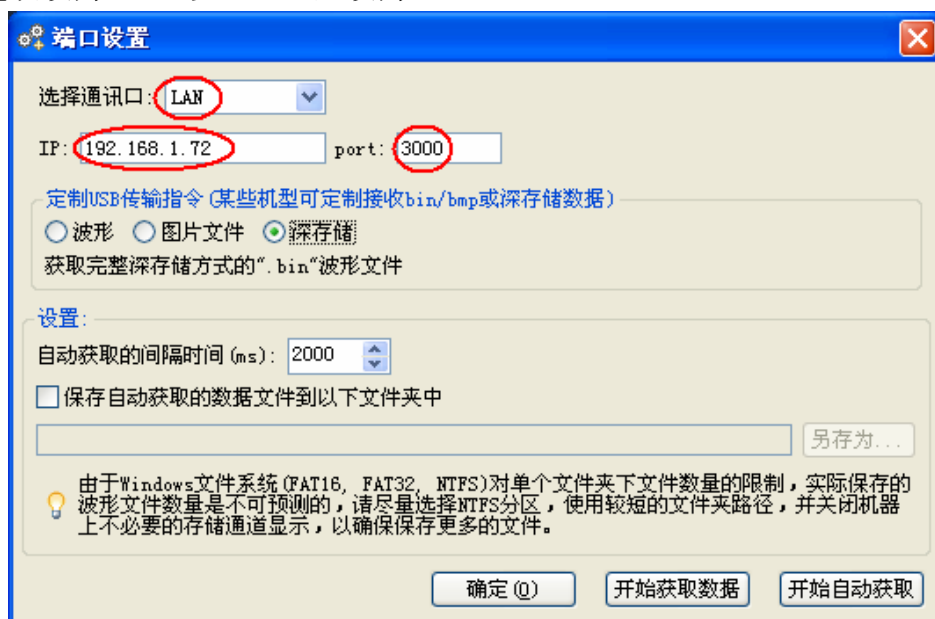
图5-51 设置上位机的网络参数
