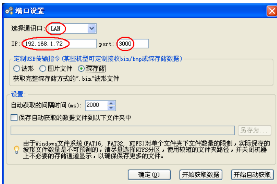
图5-48 设置上位机的网络参数
