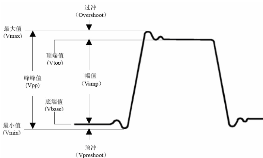
图5-55: 电压参数定义示意（顶端平整有脉冲信号）
