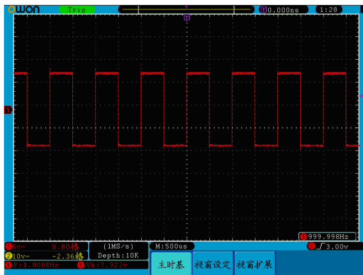
图 5-14: 主时基
