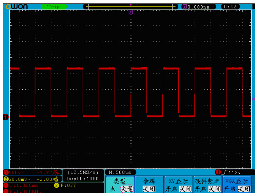
图 5-30: 矢量显示类型
