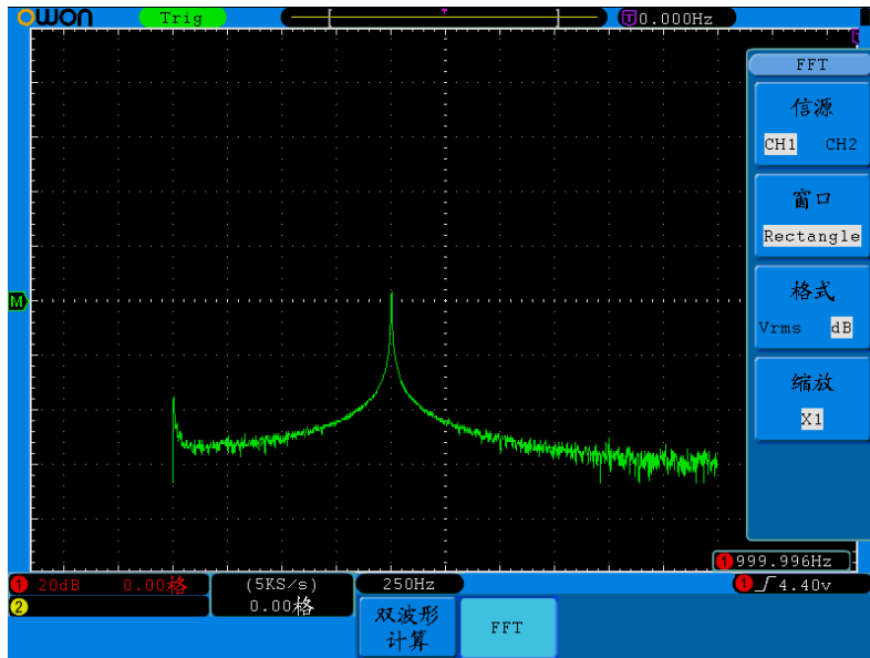
图5-10. RECTANGLE 窗
