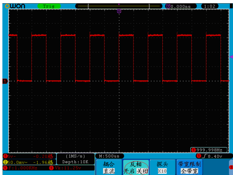
图 5-4: 未反相的波形
