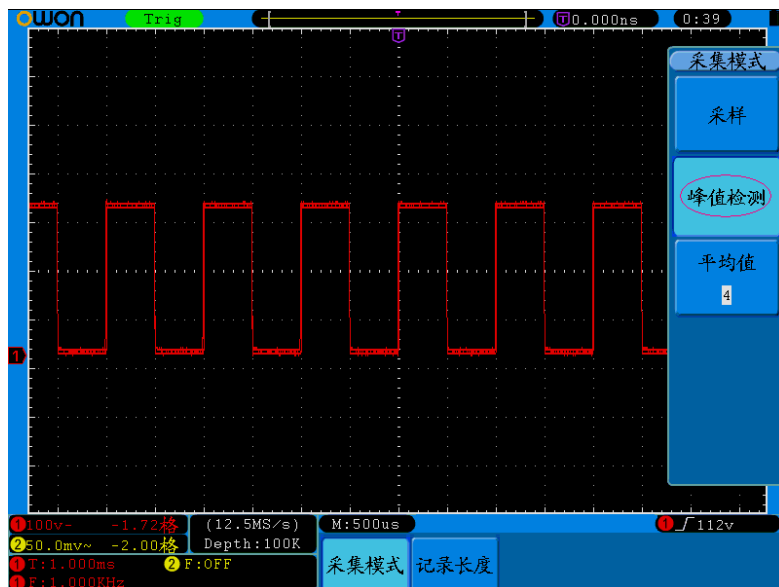
图 5-26: 峰值检测方式，可检测到方波下降沿的毛刺，噪声比较大。
