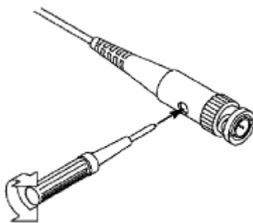
图 4-9: 探头调整
