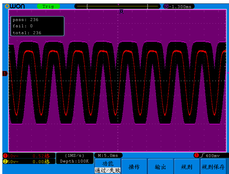
图5-44 通过/失败检测
