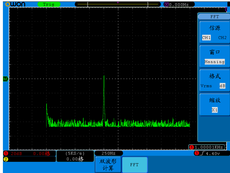
图5-9. HANNING 窗
