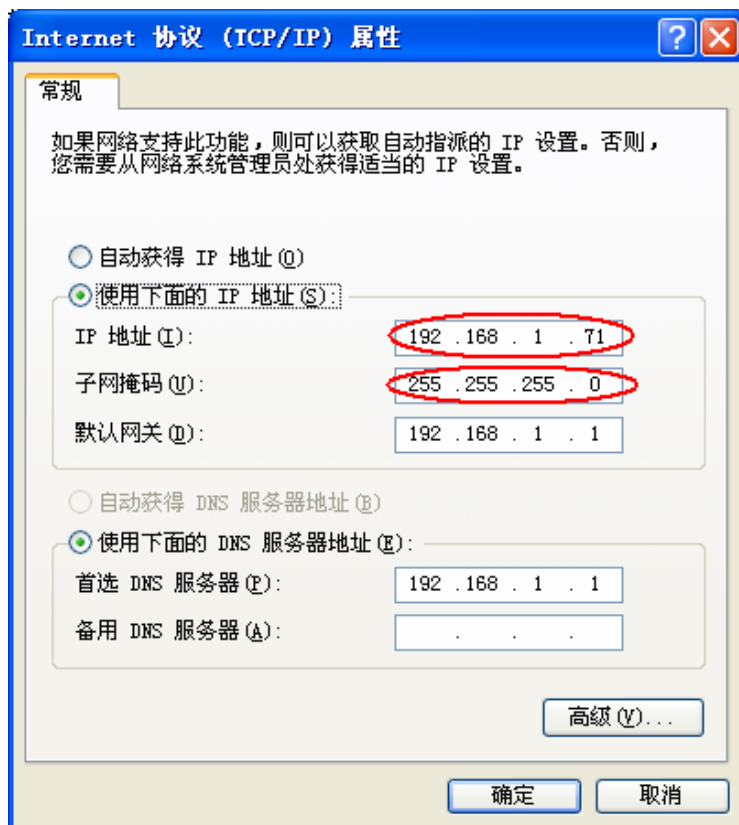
图5-47 设置计算机的网络参数
