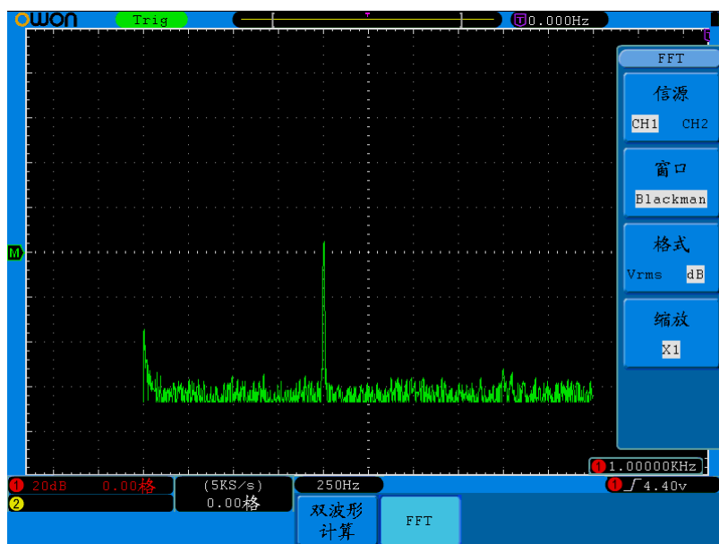
图5-8. BLACKMAN窗
