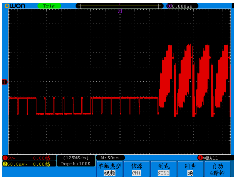
图 6-7：视频场触发波形
