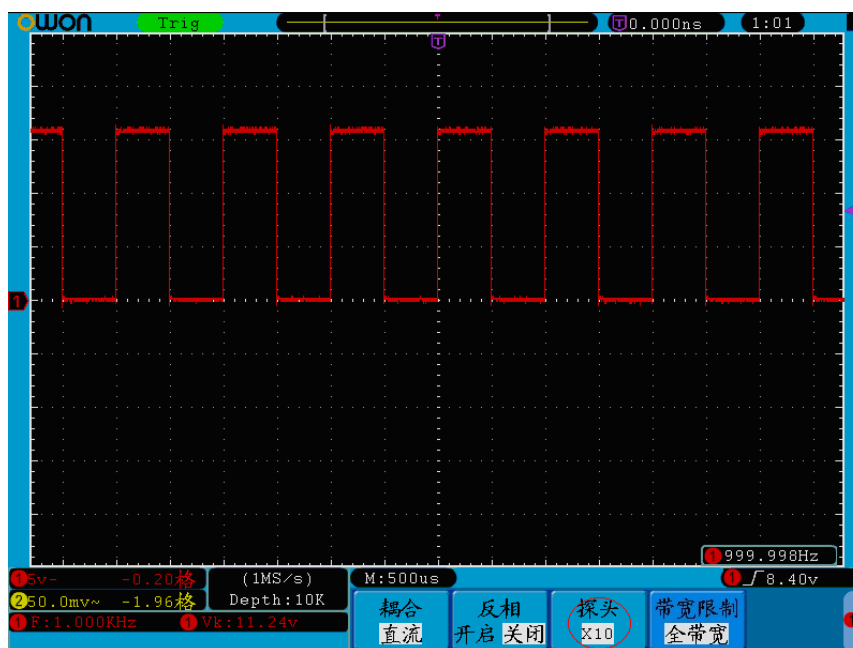
图 5-3: 调节探头比例
