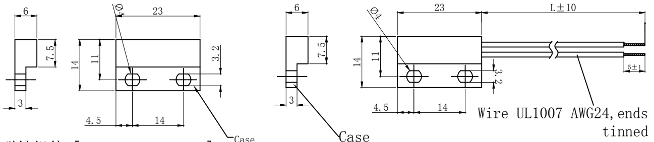
磁铁组件 [Magnet Assembly]
