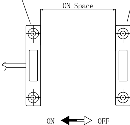
开关组件 Switch Assembly
