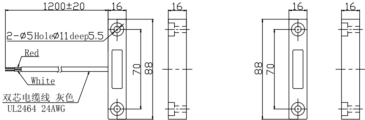
开关组件 Switch Assembly
