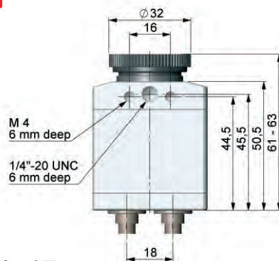
PI160尺寸图
