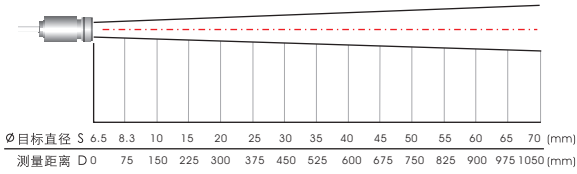
CSmicro LT, D:S=15:1
