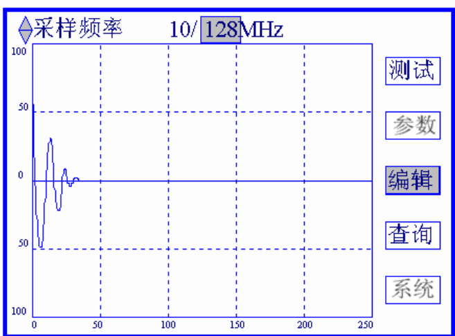
图 2C 采样频率太低: 按“ ”把波形拉开
