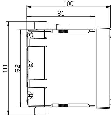
侧视图
