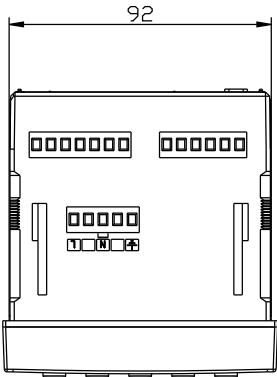
顶视图
