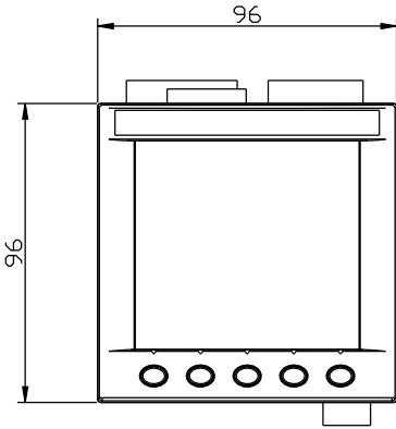
正视图
