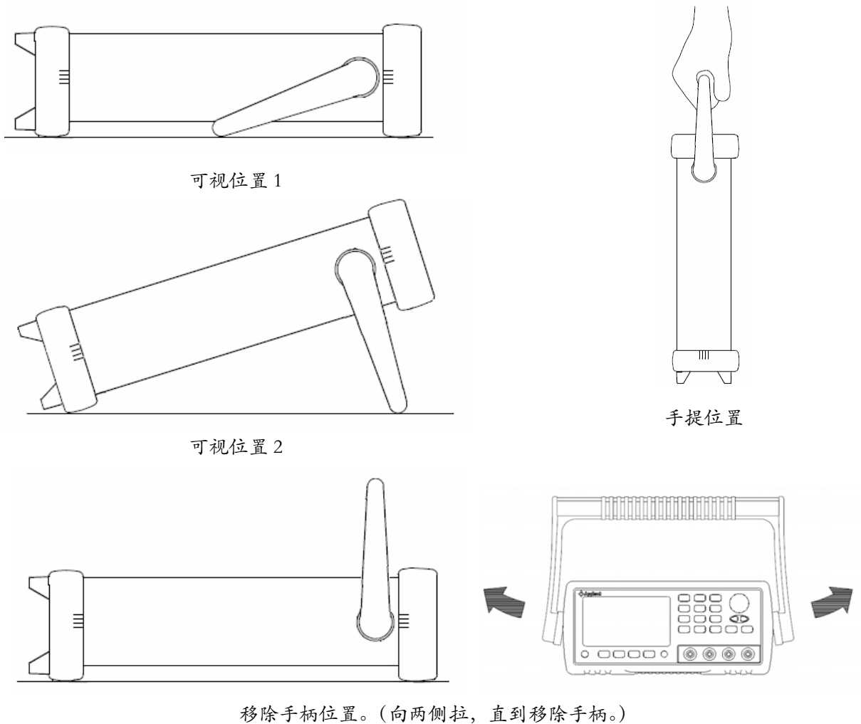
图 3-6 仪器手柄
