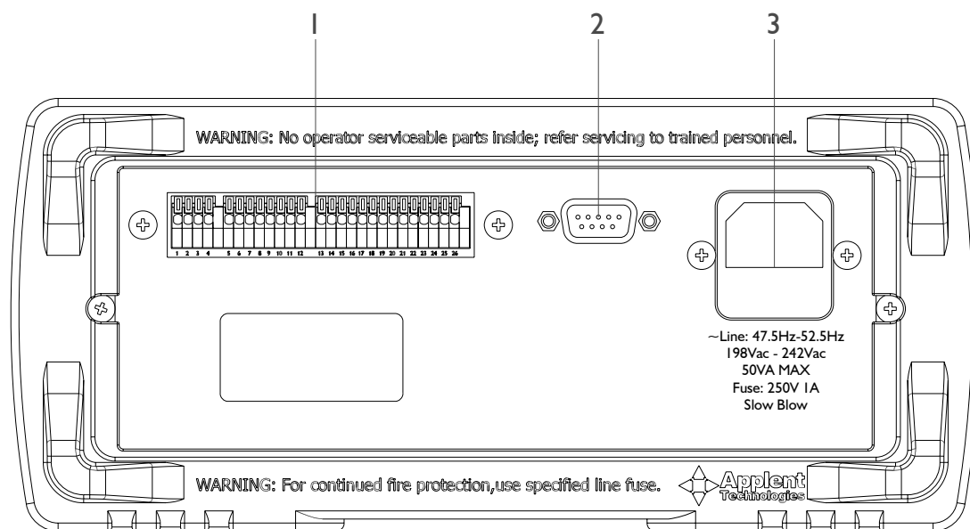
图 3-5 后面板
