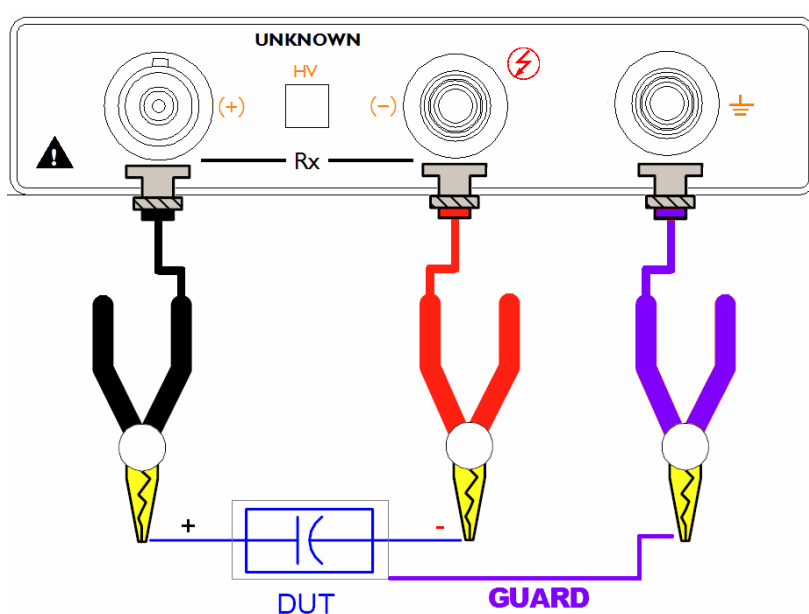
图 3-7 测试端
