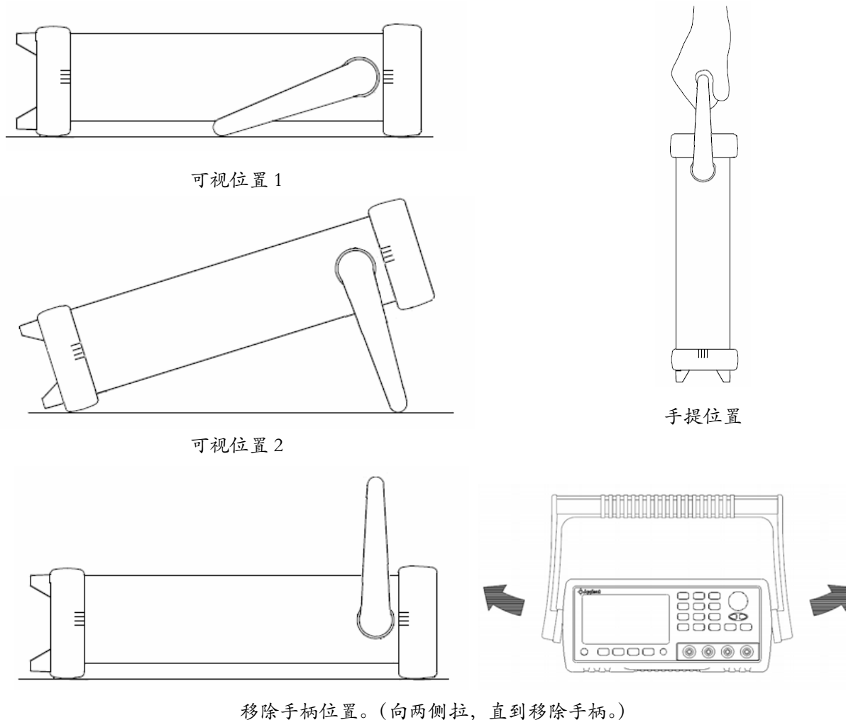
图 3-6 仪器手柄
