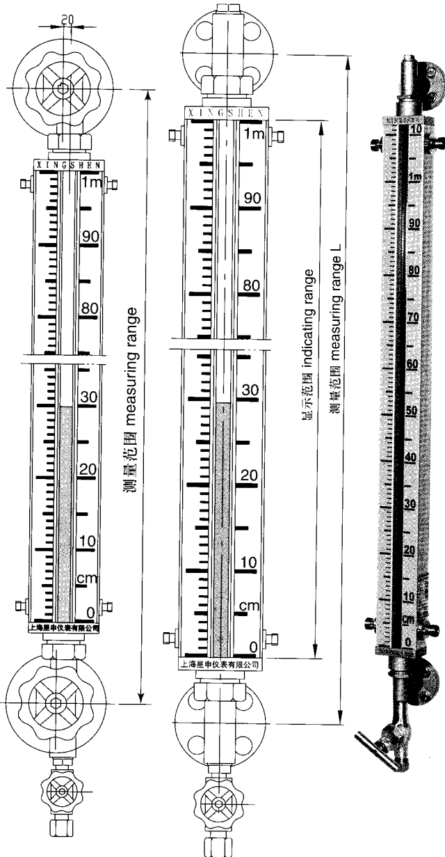
UGS-B 型
