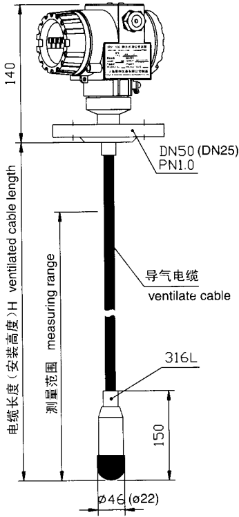
法兰安装 通用型 flange connecting, common type
