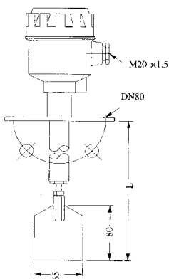
UZK-B22(轴保护管型) axis protection tube type
