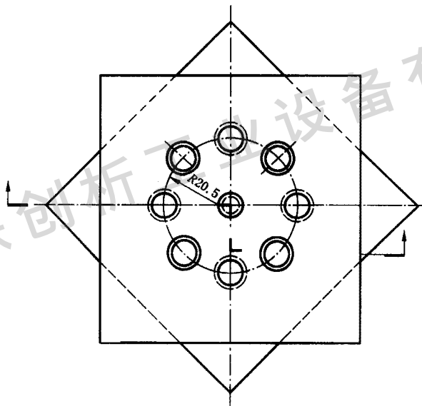
图 A.1 铆钉拉伸试验夹具
