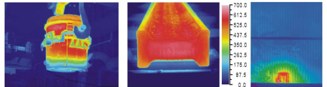
炼钢转炉
