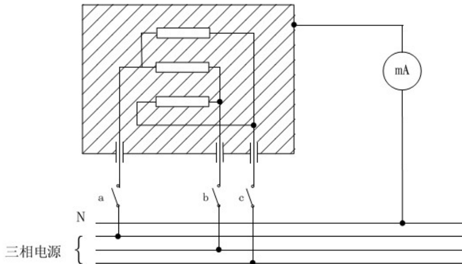
图 1-2-1 三相器具泄漏电流测量电路图
