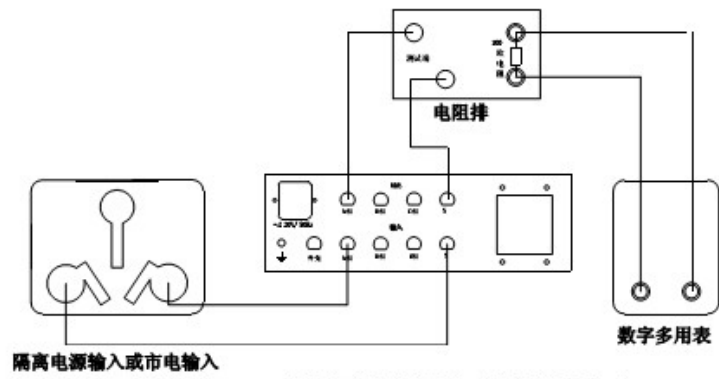
图二、泄漏电流计量接线图
