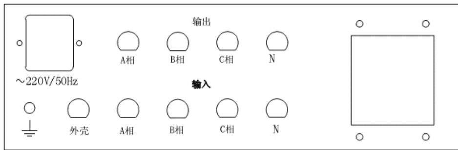
图 5-1-1 9625H 泄漏电流测试仪后面板示意图
