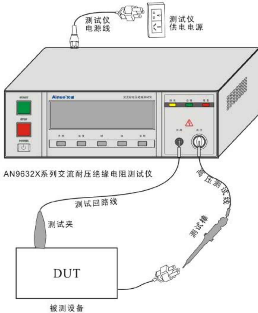
图 3.8.1 外部接线
