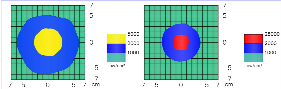
UV 辐照度强度分布图 (380mm)
