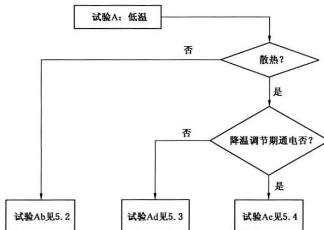
图 1 试验 A:低温试验方框图
