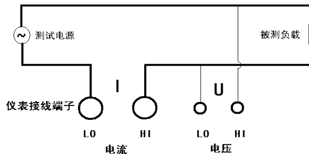
图6 测量负载接线原理图
