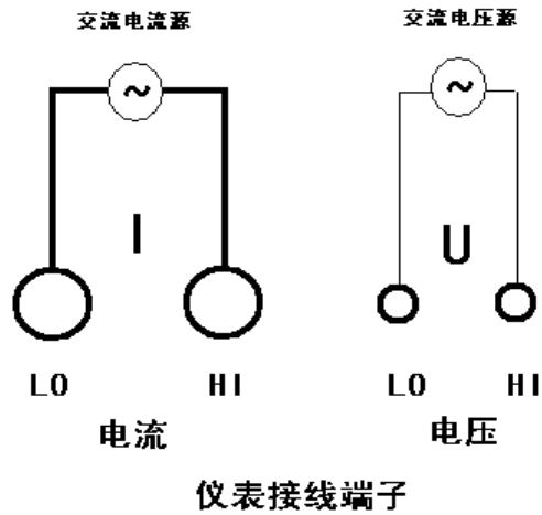
图7 检定接线图
