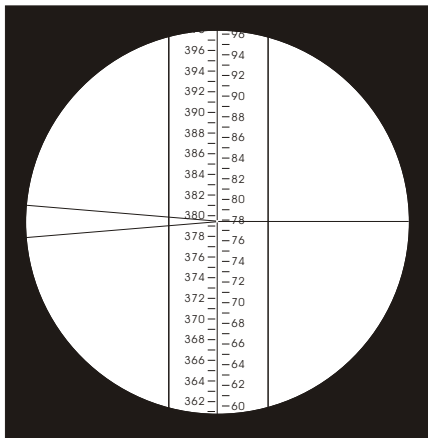
图5: DS05因瓦尺成像情况
