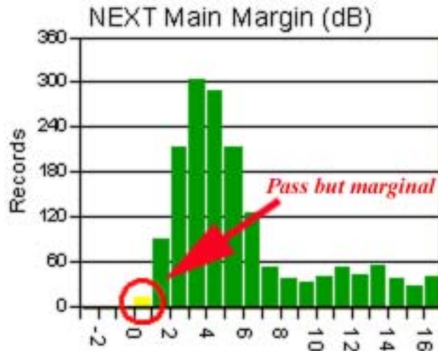
图 4：NEXT 余量柱图——正态分布
