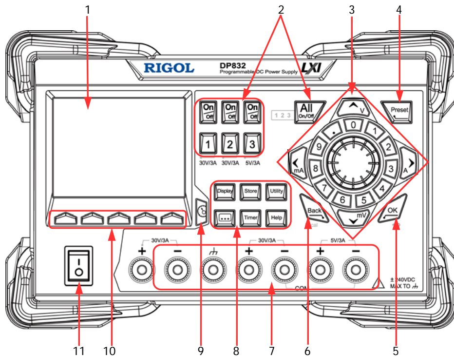
图 1-3 前面板
