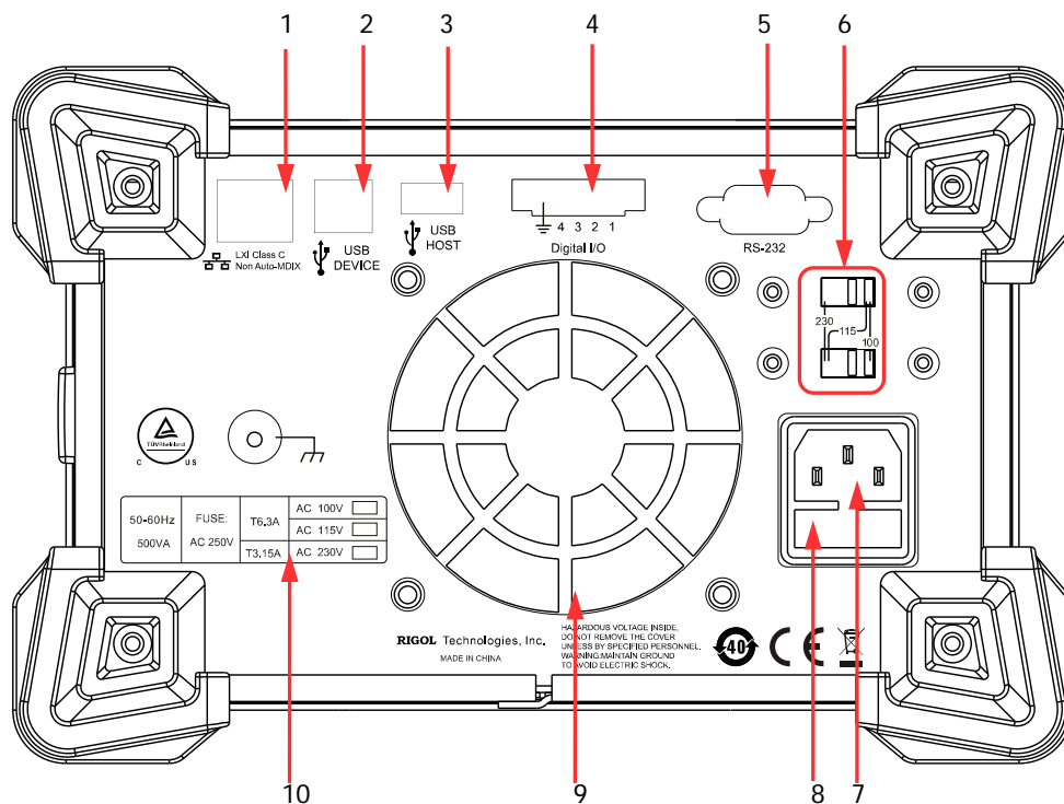
图 1-4 后面板
