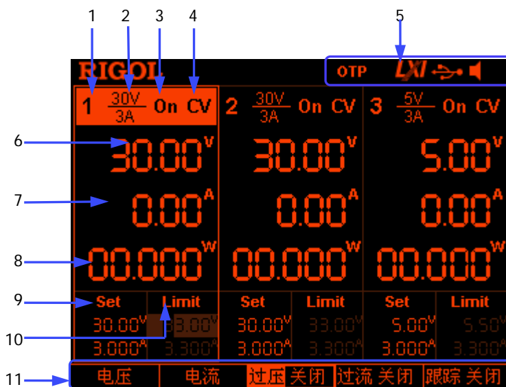
图 1-5 用户界面
