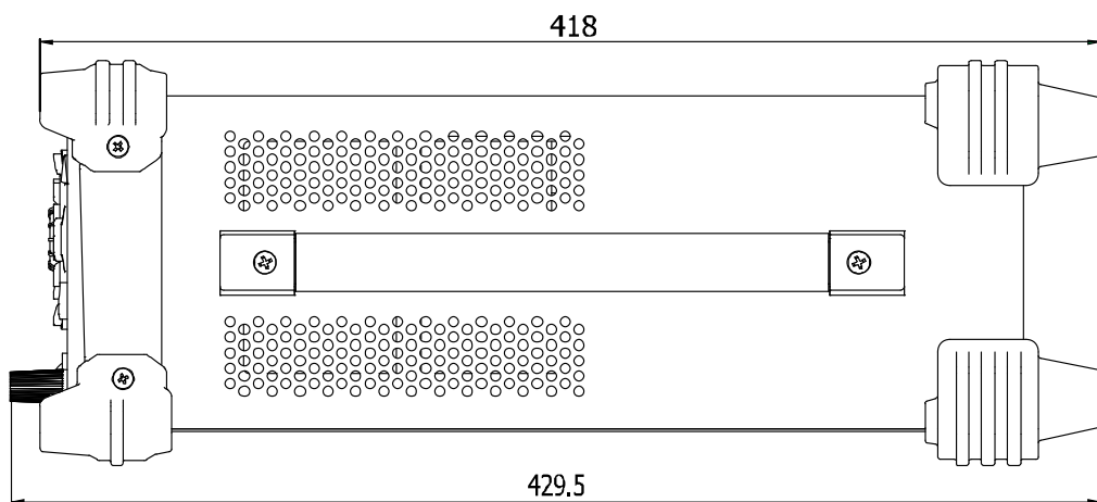
图 1-2 侧视图
