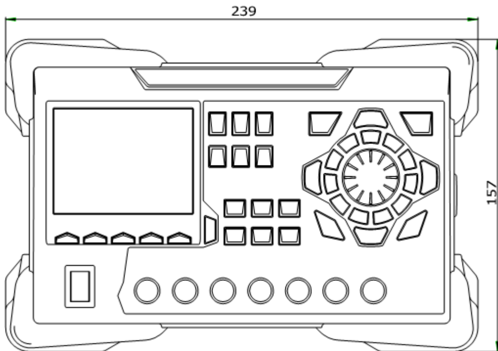
图 1-1 正视图
