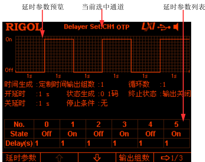
图 2-3 延时器参数设置界面
