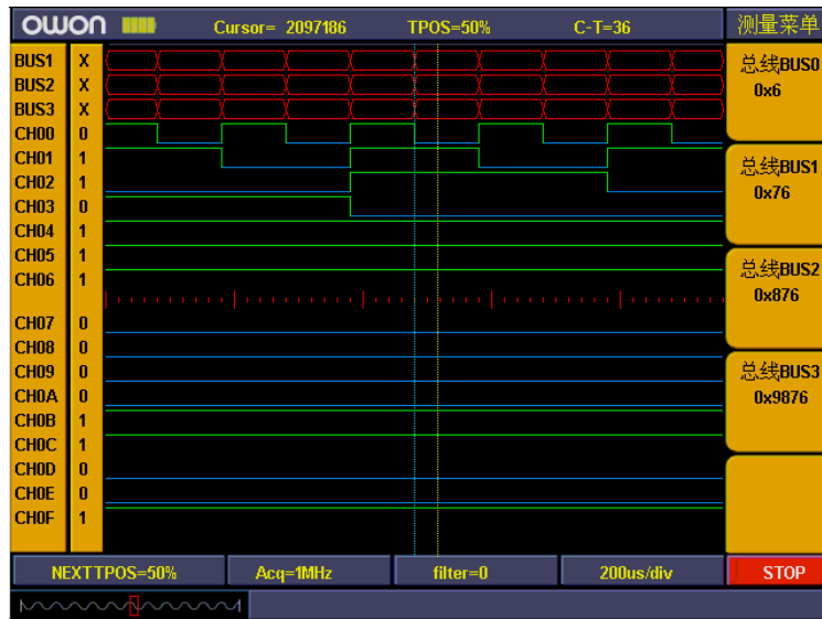
图 5-72：总线测量
