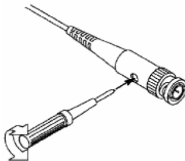
图 4-6: 探头调整
