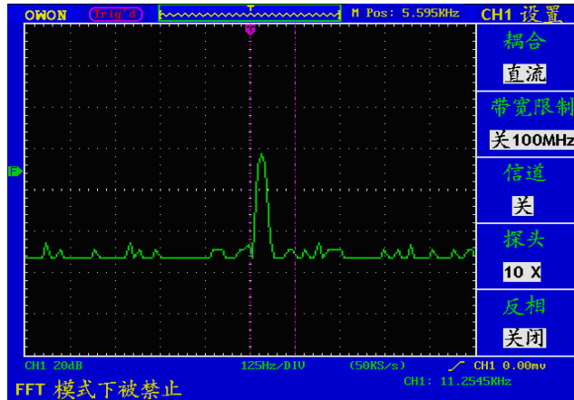
图5-4 CH1/2通道在FFT模式下被禁止
