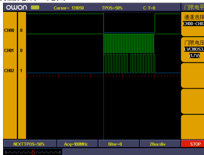
图4-17: 门限电平设置
