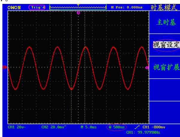
图 5-16 视窗设定
