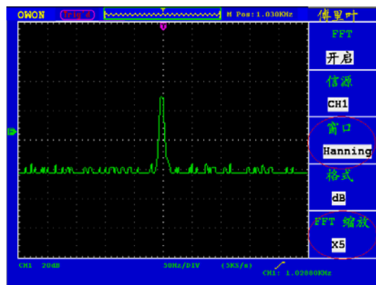
图5-10. HANNING 窗
