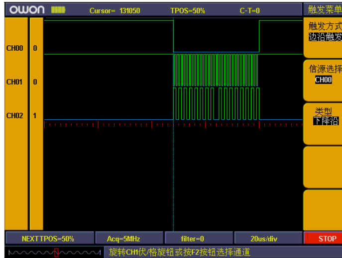
图4-16: 边沿触发设置
