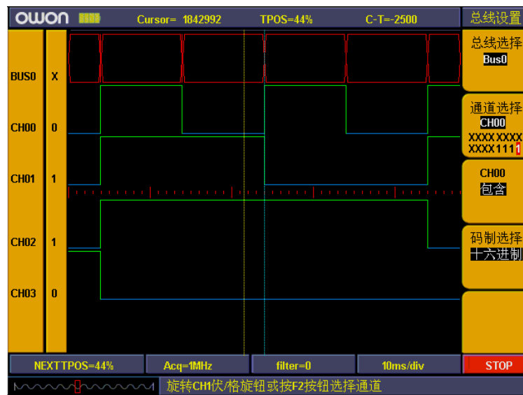
图 5-71：总线设置
