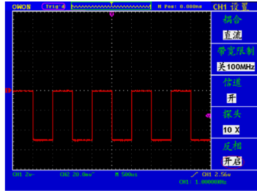
图 5-7：反相的波形
