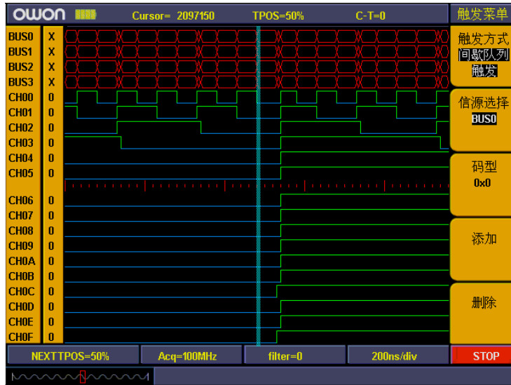
图5-63：间歇队列触发
