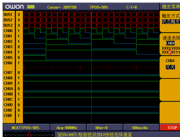
图5-59：状态触发
