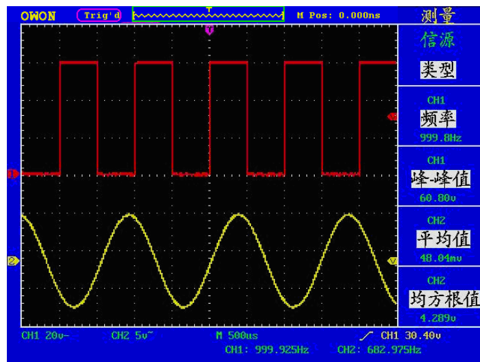
图6-1：自动测量波形
