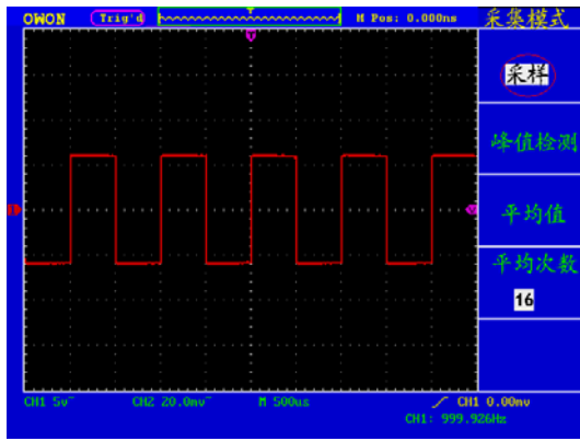
图 5-29：普通采样方式显示，检测不到毛刺。
