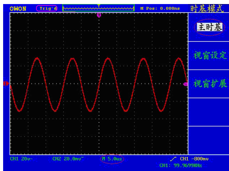
图 5-15: 主时基
