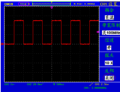
图 5-6：未反相的波形
