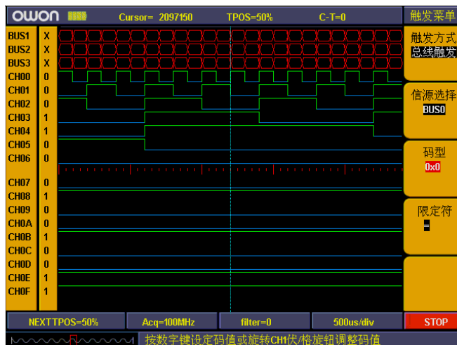
图5-57：总线触发
