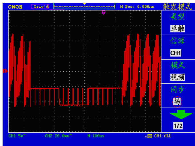
图 6-7 视频场触发波形
