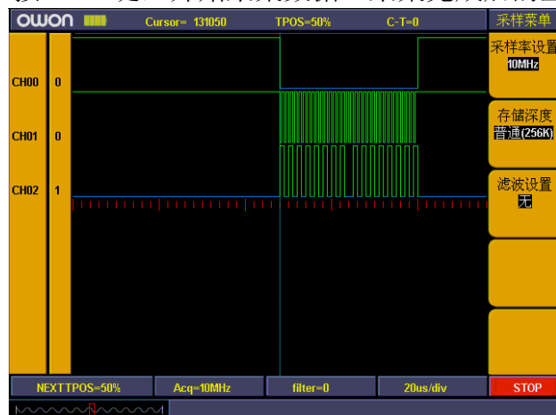
图4-19：三线SPI信号
