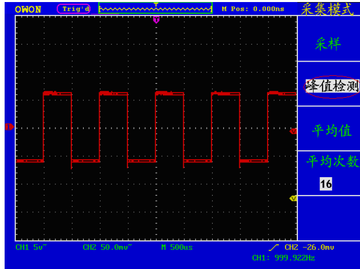
图6-4 含噪声信号的波形
