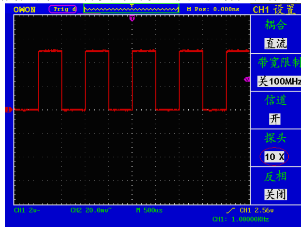
图 5-5：调节探头比例
