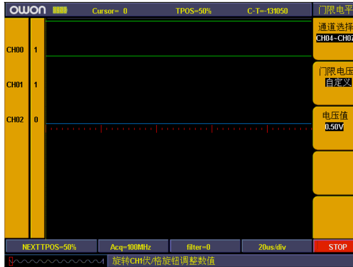
图 5-67：门限电平自定义设置
