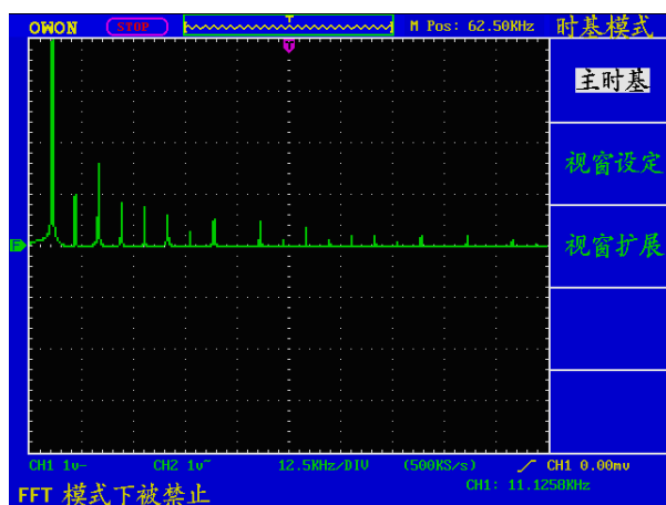
图5-17 FFT模式下视窗设定被禁止
