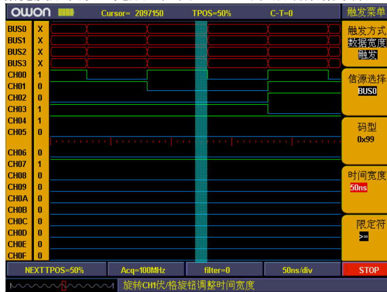
图5-65：数据宽度触发
