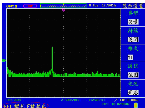
图5-36. FFT模式禁止更改YT格式
