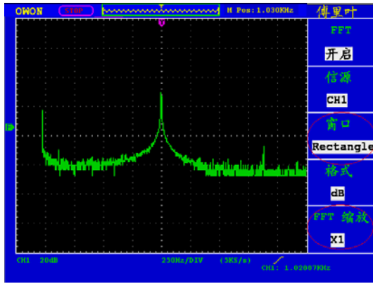
图5-11. RECTANGLE 窗
