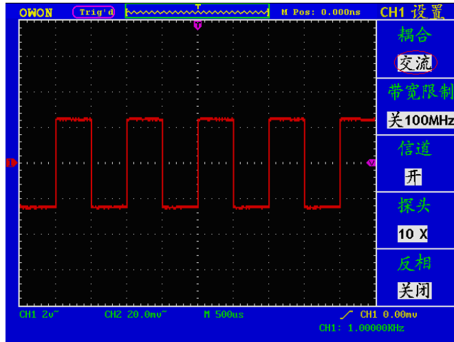
图5-2: 交流耦合波形图
