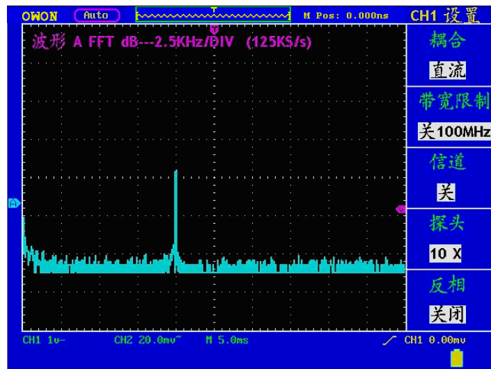
图5-39：FFT波形存储
