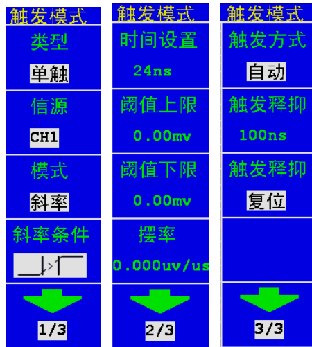
图 5-22 斜率触发菜单
