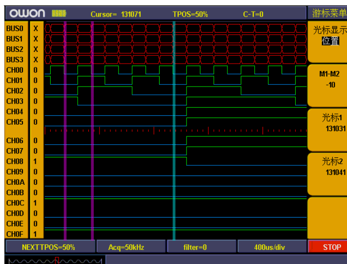
图 5-81 光标位置测量
