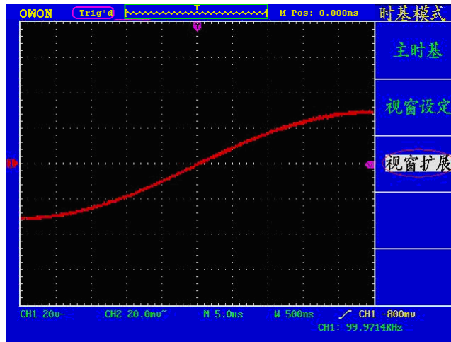
图 5-18 视窗扩展
