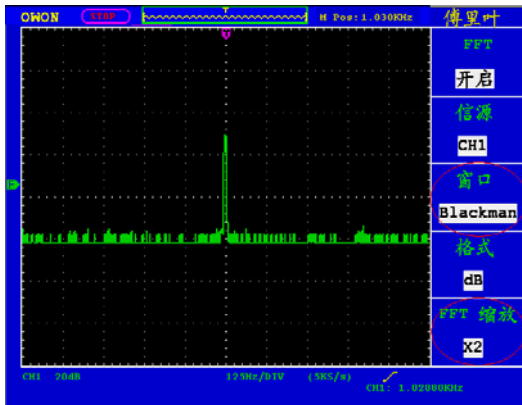
图5-9. BLACKMAN窗
