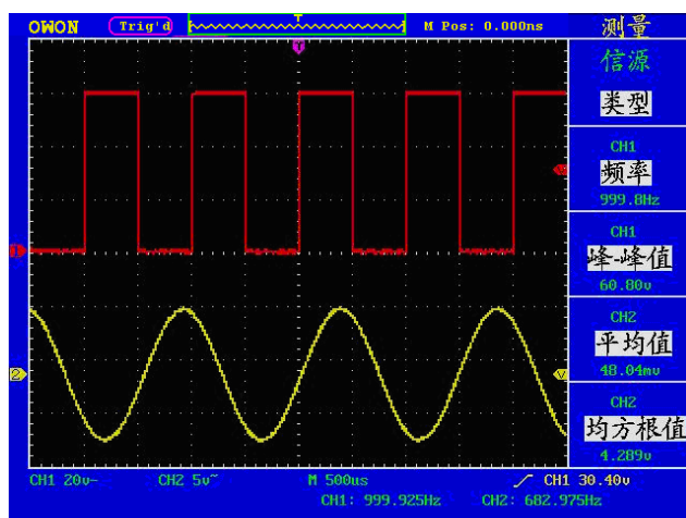
图5-44：自动测量
