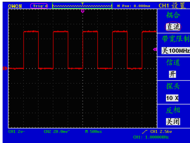
图 5-3: 直流耦合波形图
