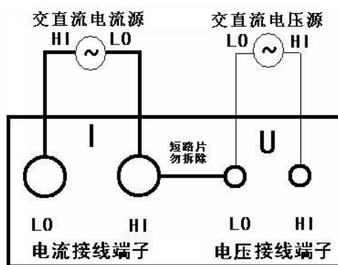
(电压源与电流源共地)
