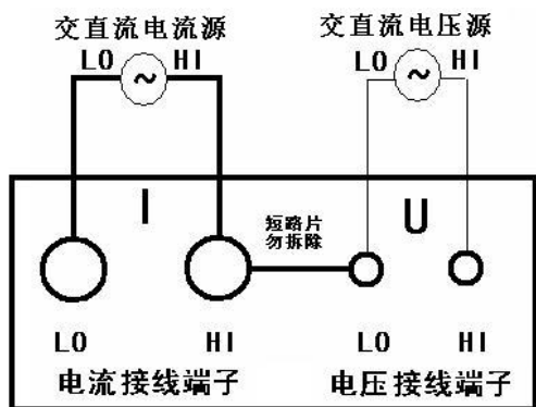
(电压源与电流源相互隔离)
