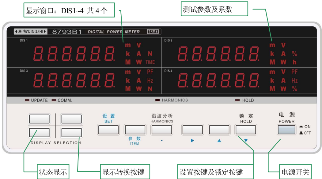
图 2 仪表前面板示意图
