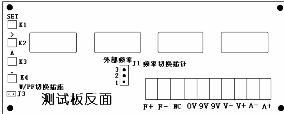
仪表反面接线位置图
