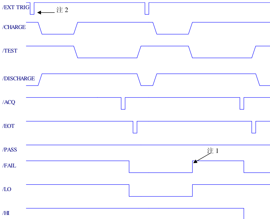
图 7-2 SEQ.TEST 时序
