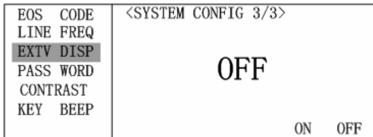
图 3-45 EXTV DISP
