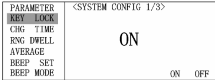
图 3-30 键锁设置
