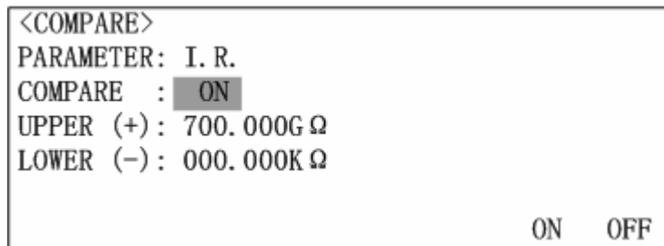
图 3-21 COMPARE 页选项
