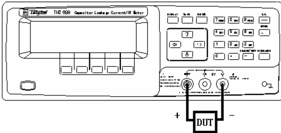
图 3-1 被测件连接图
