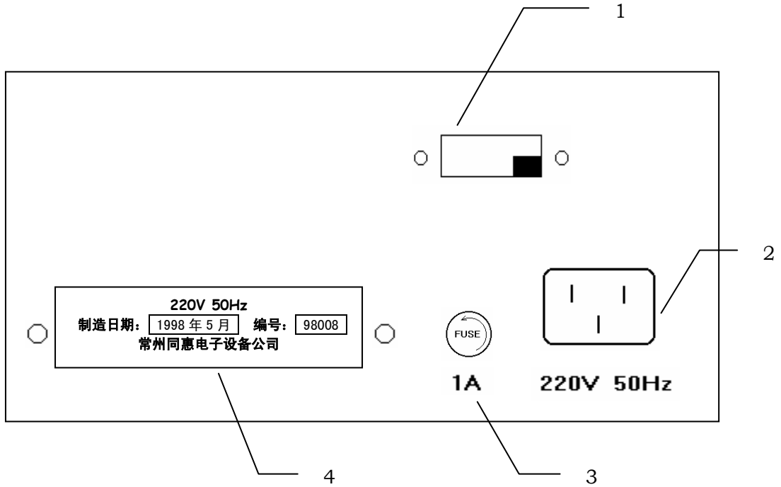
图 1-2 后面板图
