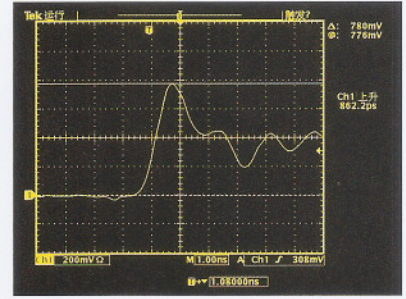
电流前沿波形
