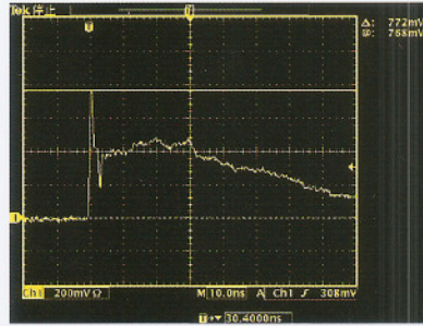
放电电流波形
