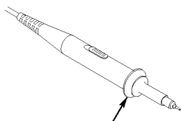
手指防护装置
