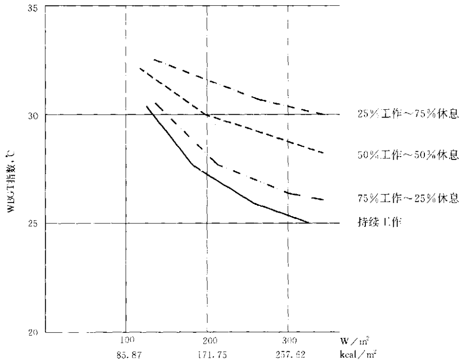
图 B1 各种劳动/休息时间的 WBGT 参考值的曲线
