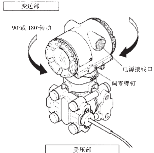
图 4.5.1 变送部的转动
