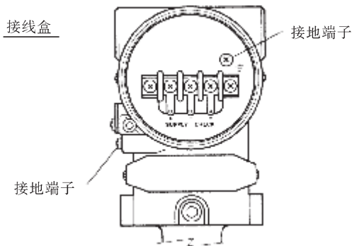
图 5.5 接地端子
