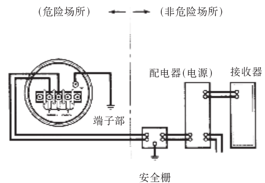
图 5.4.1b 变送器与配电器的连接
