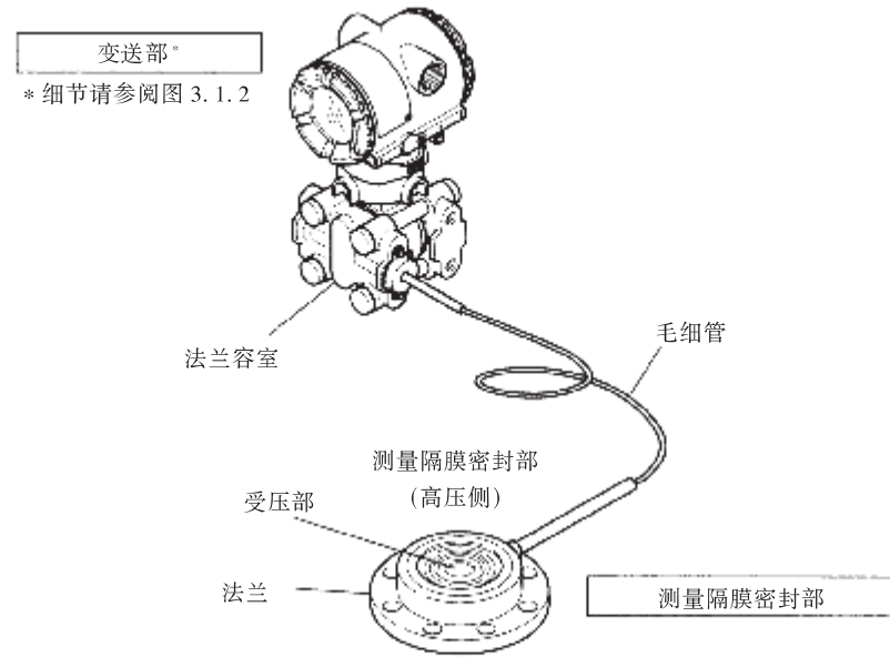
图 3.1.1 各部件名称(EJA438W)
