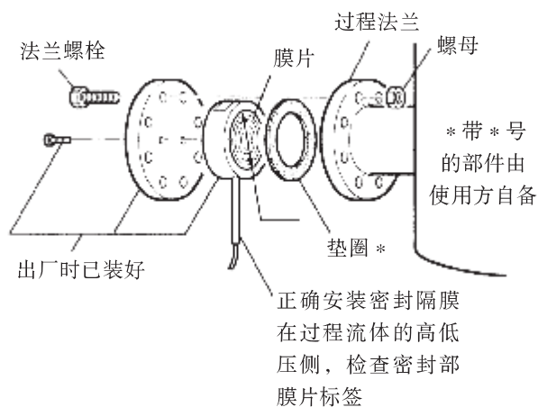
图 4.1 远传法兰隔膜密封部的安装
