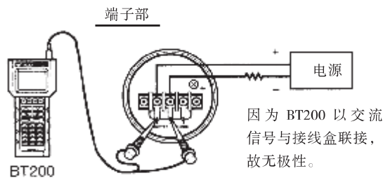
图 5.3.3 BT200 的连接
