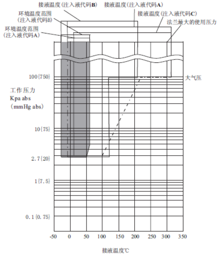
图 1 工作压力和接液温度
