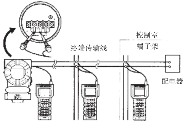
图 7.1.1 BT200 的连接
