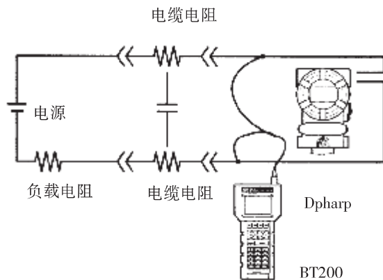
图 7.1.2 通信线要求
