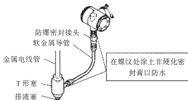
图 5.4.2b 配线用隔爆密封接头
