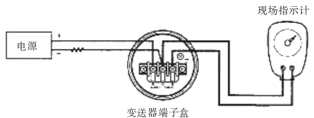
图 5.3.2 外接指示计连接
