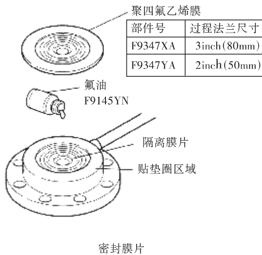
图 4.4.1 聚四氟乙烯膜片的安装
