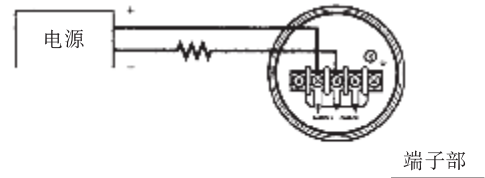
图 5.3.1 电源连接
