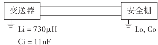
图 2.5 安全栅连接图
