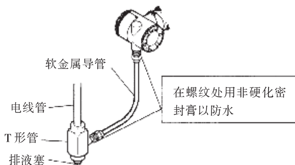
图5.4.2a 配线用金属软管
