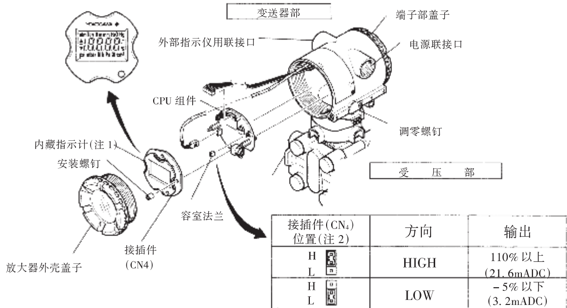
图 3.1.1 各部件名称(EJA438W)
