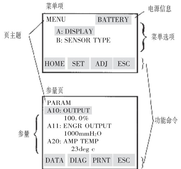
图 7.2.1 BT200 键面图
