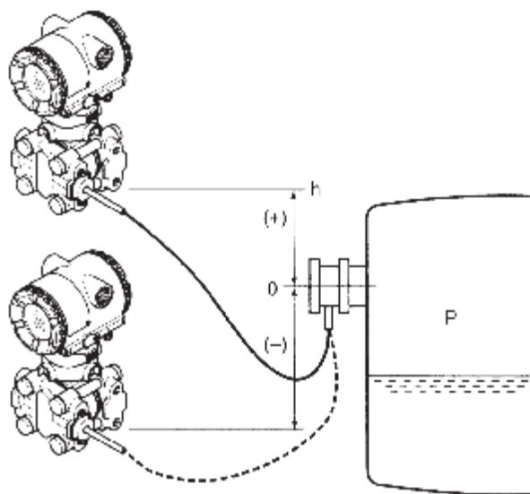
图 4.3.2 在液罐上的安装实例(注意安装)
