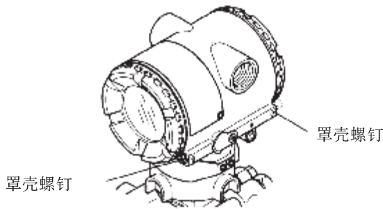
图 8.4.1 罩盖螺钉
