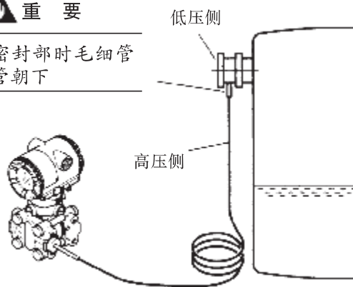
图 4.2 液罐安装实例
