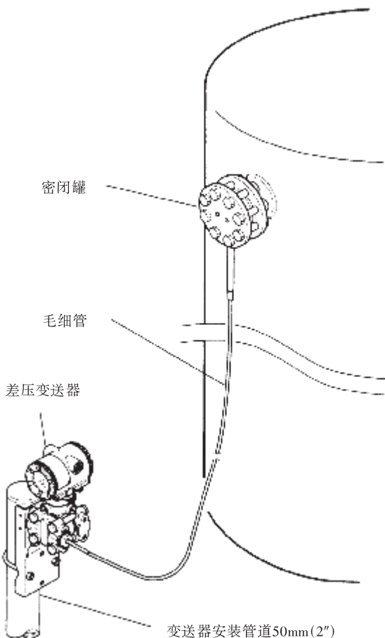
图 6.1 密封容器的液位测量
