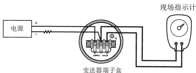
图 6.3.2 外接指示计连接
