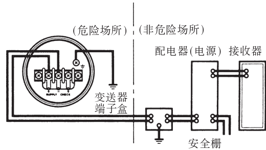
图 6.4.1b 变送器与配电器的连接
