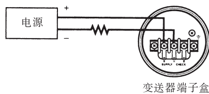
图 6.3.1 电源连接
