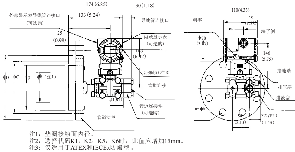
法兰尺寸: 3inch(80mm, DN80)
