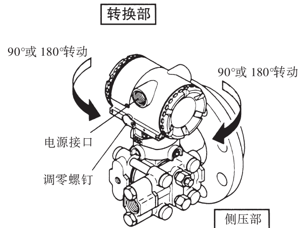
图 4.2 转换部的旋转
