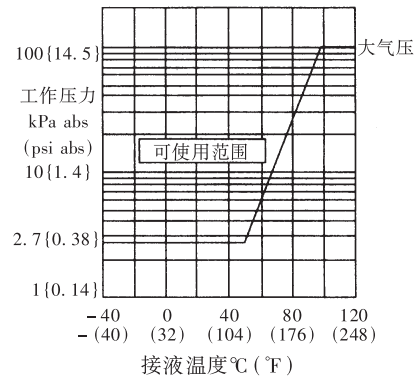
图 1 工作压力和环境温度关系图
