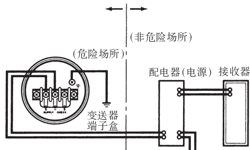
图 6.4.1a 变送器与配电器的连接
