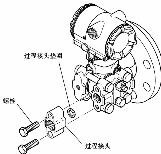
图 9.4.2 过程接头垫圈的更换
