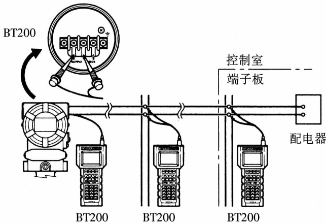
图 8.1.1 BT200 的连接
