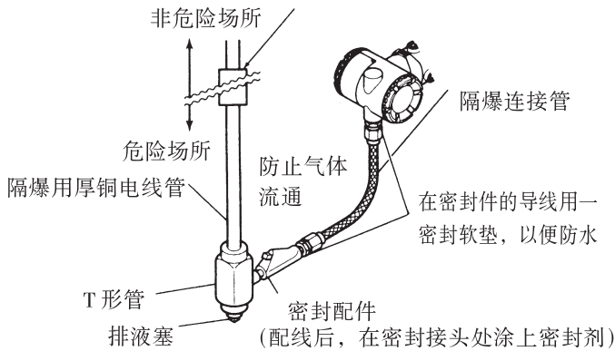
图 6.4.2c 使用隔爆金属导线管配线
