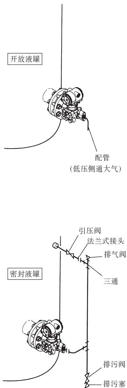
图 5.2 配管例
