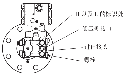
图 5.1 膜合组件的 H、L 标识场所
