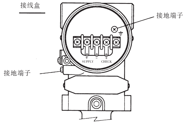
图 6.5 接地端子
