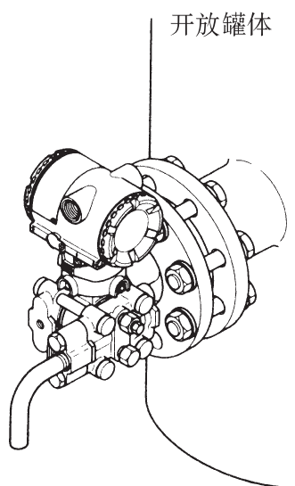
图 7.1 液位测量
