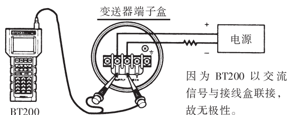
图 6.3.3 BT200 的连接
