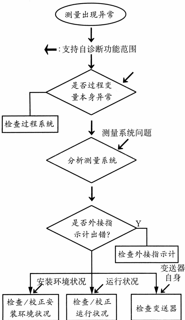
图 9.5.1 基本流程及自诊断
