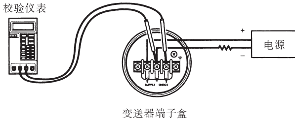
图 6.3.4 校验仪表连接
