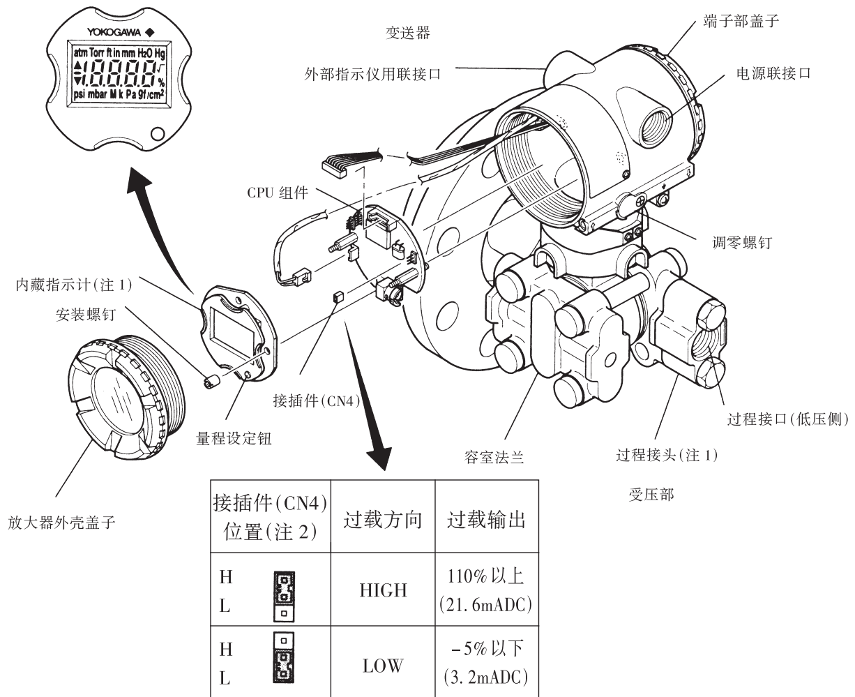
图 3.1.1 各部分和名称
