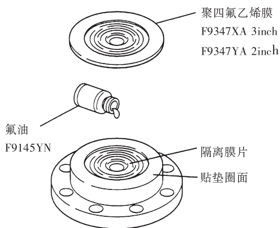
图 4.3 聚四氟烯膜片的安装
