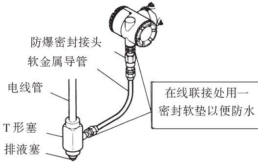
图 6.4.2b 配线用隔爆密封接头
