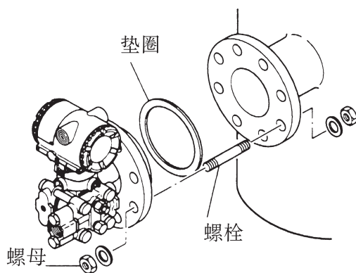
图 4.1 变送器的安装
