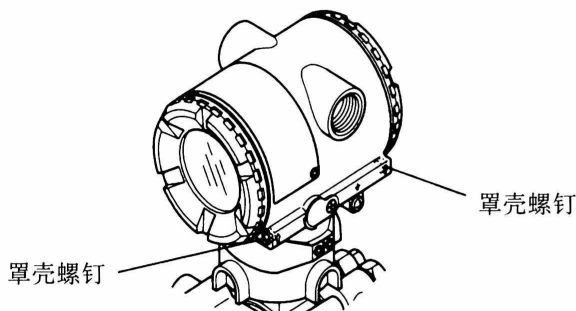
图 9.4 罩盖螺钉
