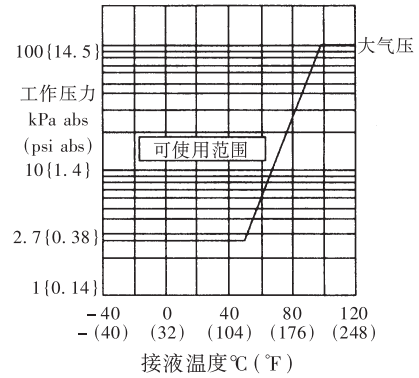
图 1 工作压力和环境温度关系图
