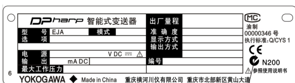
图 2.2 铭牌
