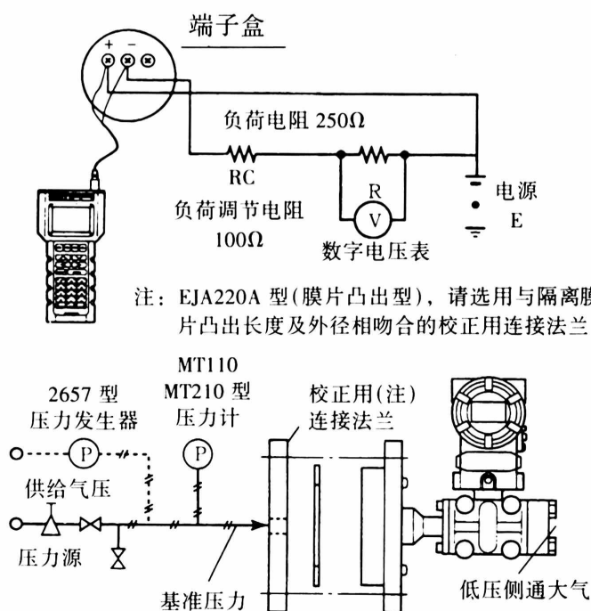
图 9.3.1 仪表连接
