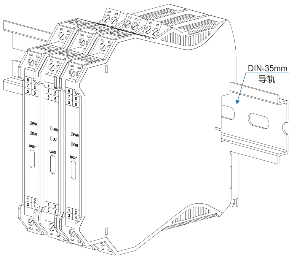
图 4 标准导轨卡式安装示意图
