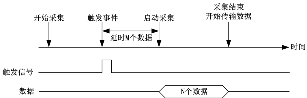
图 4-9-2-6 硬件延时触发
