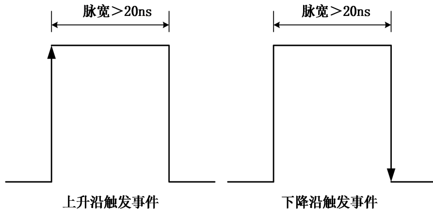
图 4-8-8 脉宽最小值图
