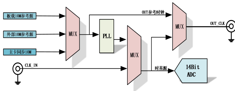
图 4-7-1 时基源框图
