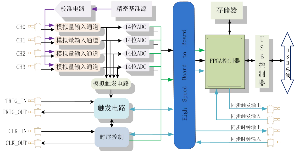
图 3-1-1 USB8504\8514 系统框图
