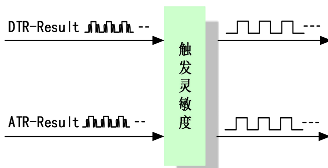
图 4-8-2 触发灵敏度
