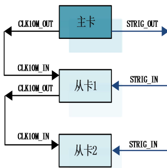
图 4-10-1 主从卡级联
