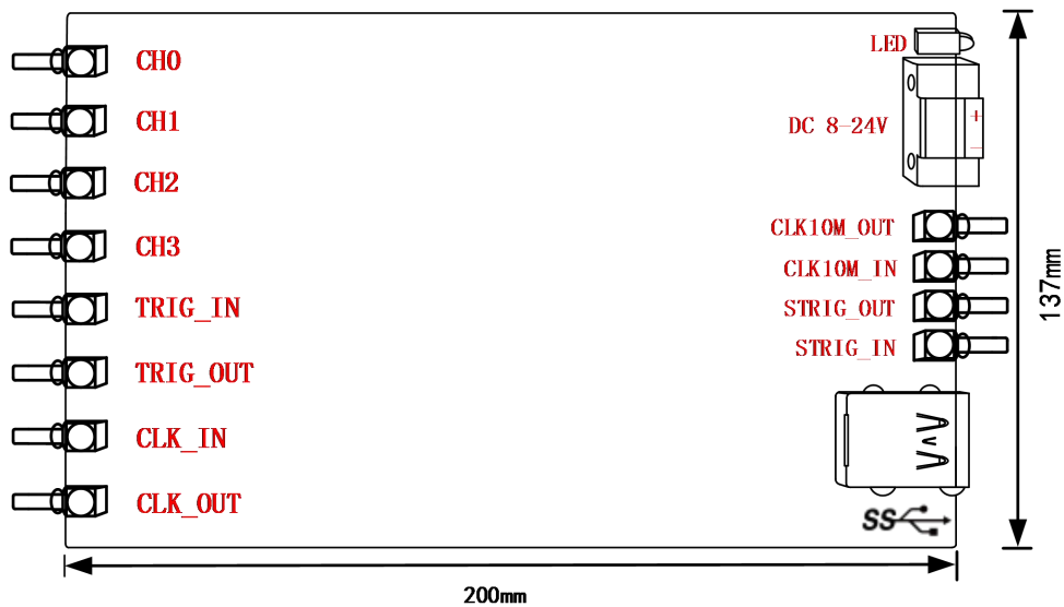
图 3-2-1 USB8504\8514 板卡尺寸图
