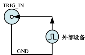
图 4-8-7 DTR 触发信号连接
