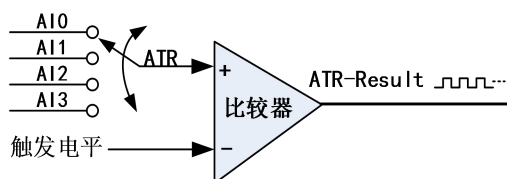
图 4-8-5 比较器
