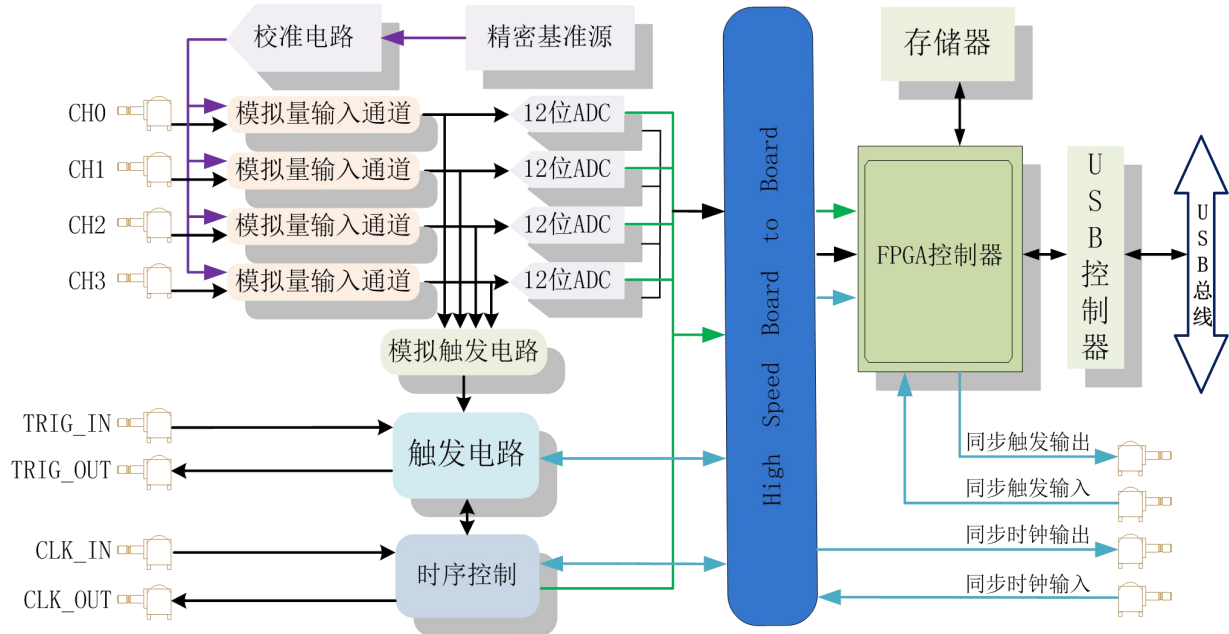
图 3-1-1 USB8502\8512 系统框图
