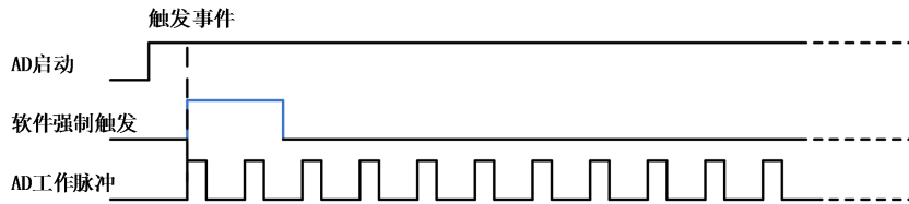
图 4-8-3 AD 软件触发
