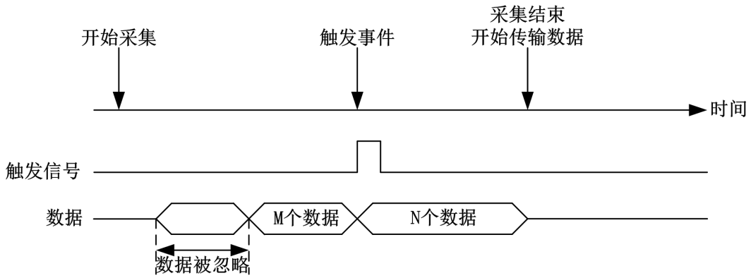
图 4-9-2-2 中间触发
