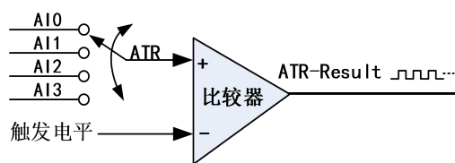
图4-8-5 比较器
