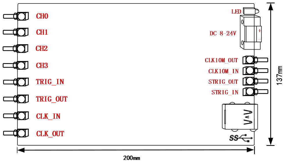
图 3-2-1 USB8502\8512 板卡尺寸图
