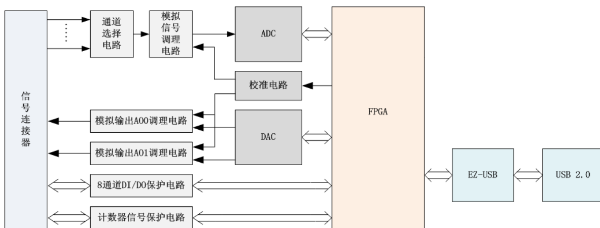
图 2-2-1 USB5621U 系统框图
