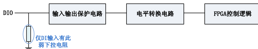
图6-1-1 数字量输入输出功能框图
