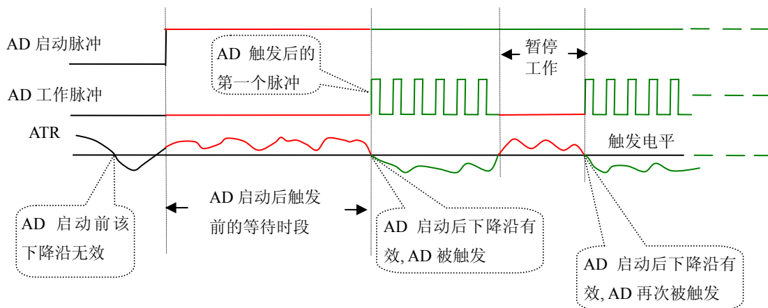
图 7.4 低电平触发
