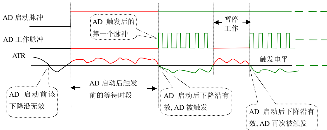
图 7.4 低电平触发
