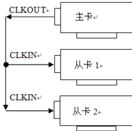
多卡级联的连接方法
