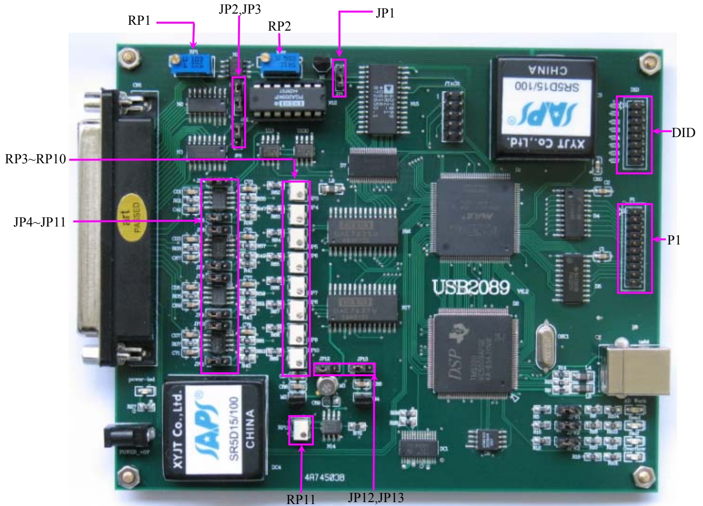
图 2.1 USB2089 板图
