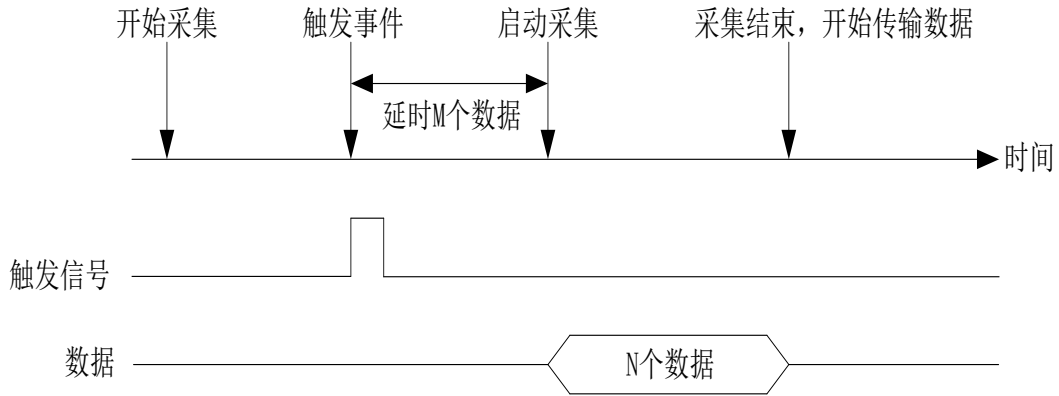
图 8-2-4 硬件延时触发
