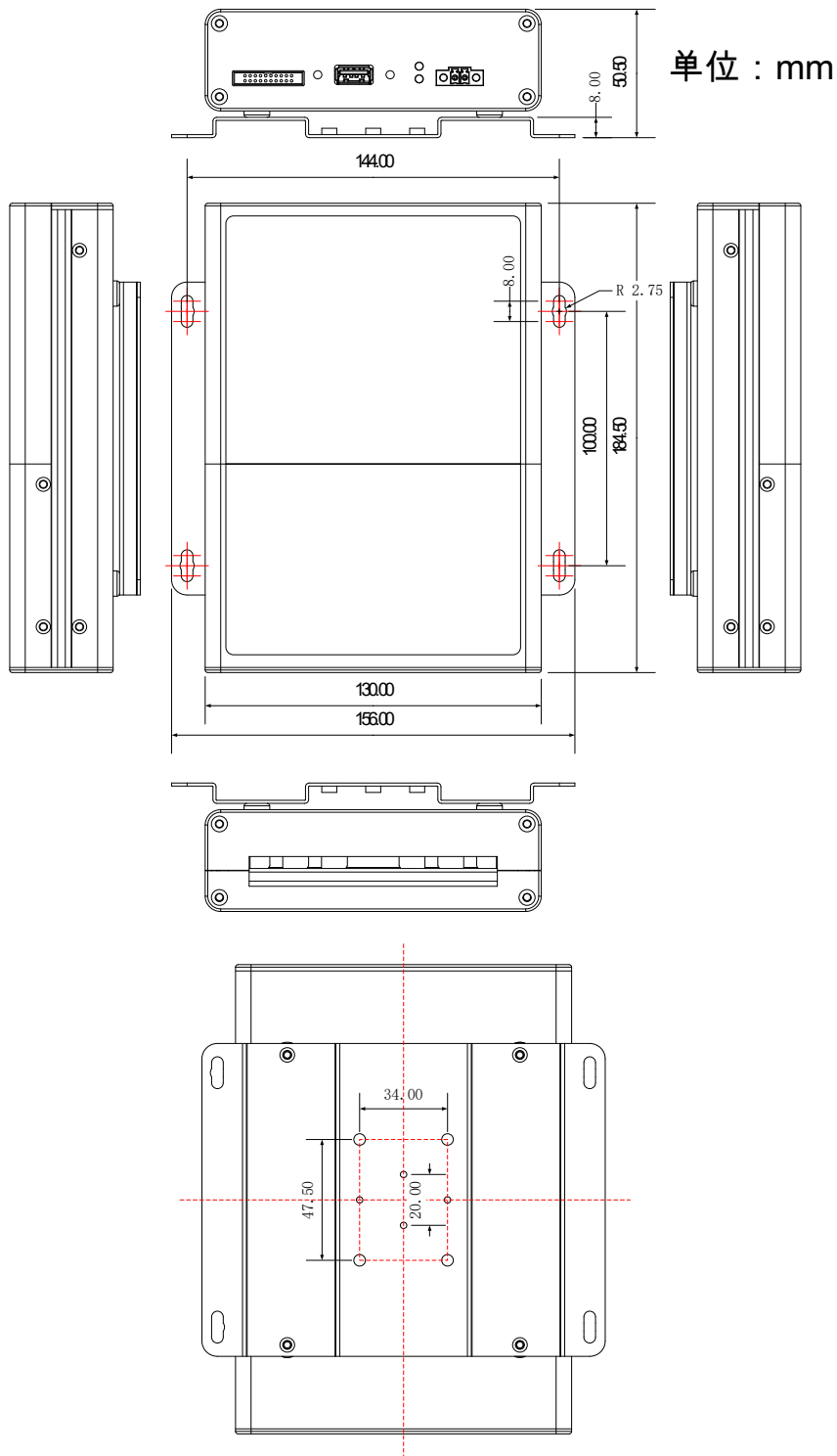
图 3-2-1 USB287X/XA/XB/XC-D 外壳尺寸图
