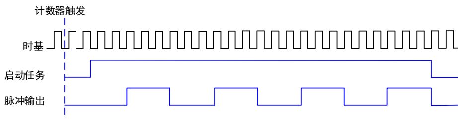
图 6-8-3 有限脉冲序列生成
