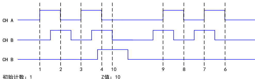
图 6-7-6 Z 索引
