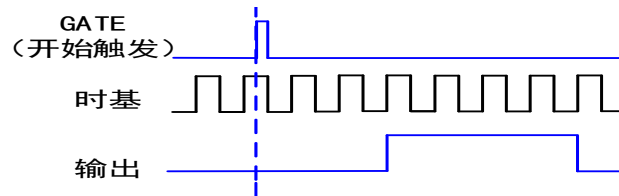
图 6-8-2 具有启动触发的单脉冲生成
