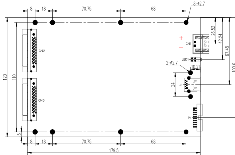
图 3-2-3 USB287X/XA/XB/XC 板卡内部尺寸图
