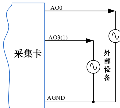
图5-2-1 AO模拟量输出连接
