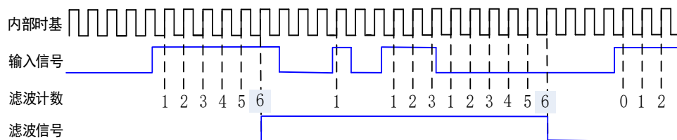
图 6-9-1 脉冲输出
