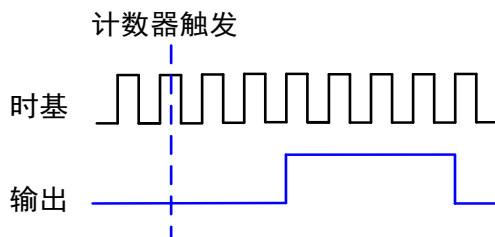
图 6-8-1 单脉冲生成
