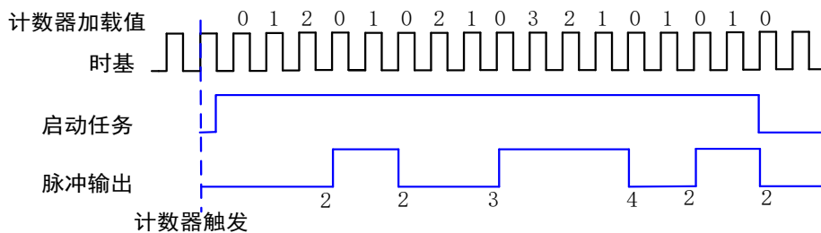
图 6-8-7 有限隐式缓冲脉冲序列生成
