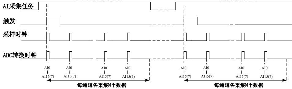
图 4-7-2 有限点采样
