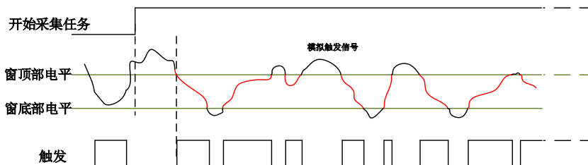
图8-3-7 模拟窗触发--入窗
