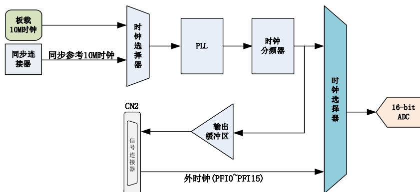
图 4-6-1 AI 时钟结构框图
