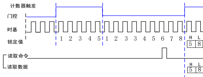
图 6-4-1 单（按需）脉冲测量
