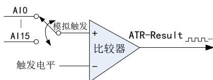
图8-3-4 模拟触发比较器
