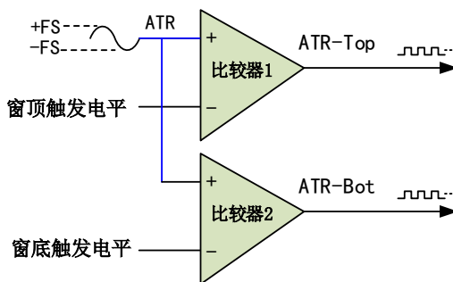
图8-3-6 比较器
