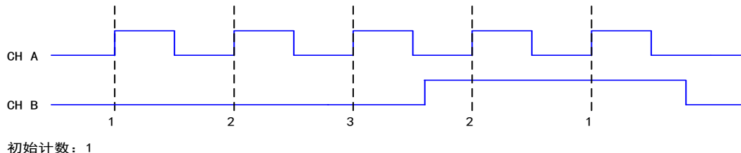
图 6-7-5 单脉冲编码
