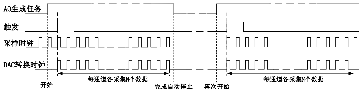
图5-7-2 内、外时钟有限点采样
