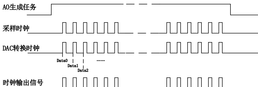
图 5-6-2 内时钟时序图
