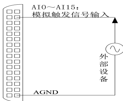
图8-3-3 模拟触发连接方法
