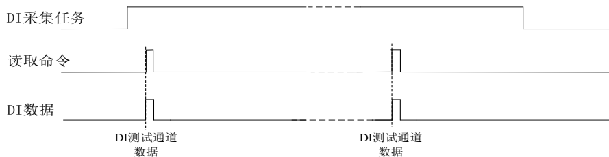
图7-5-1 按需单点采集
