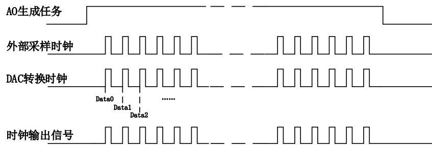
图 5-6-3 外时钟时序图
