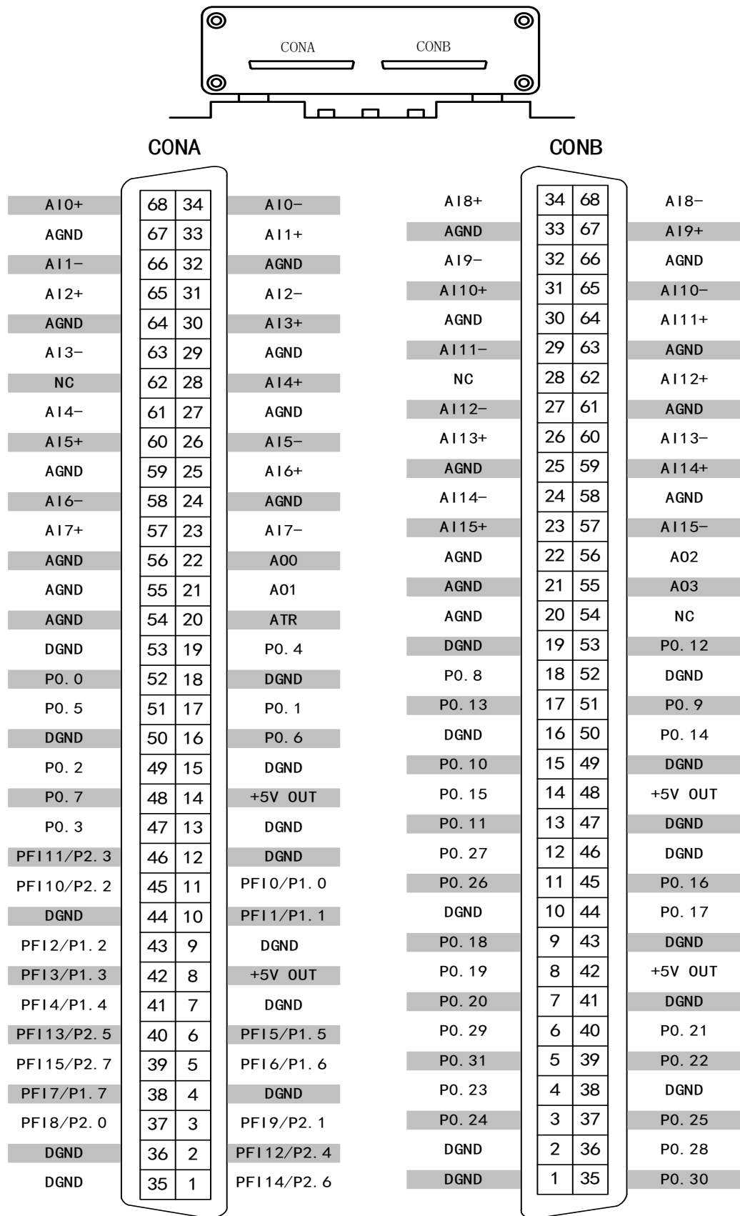
图3-3-2 VHDCl连接器管脚定义
