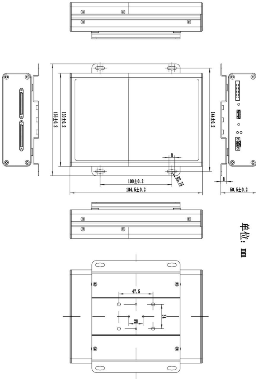
图 3-2-2 USB287X/XA/XB/XC-V 外壳尺寸图
