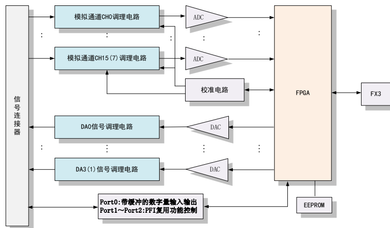
图2-2-1 USB287X/XA/XB/XC系统框图
