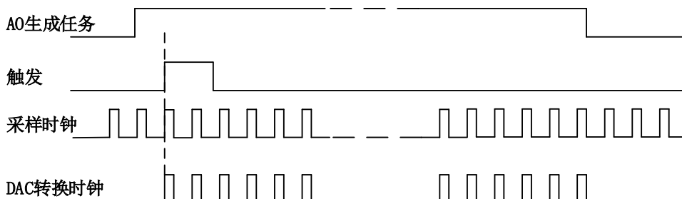
图5-7-3 内、外时钟连续采样
