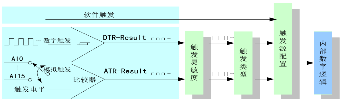
图 8-1-2 模拟触发源选择
