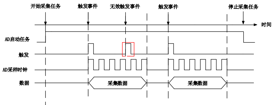
图 8-2-6 重触发
