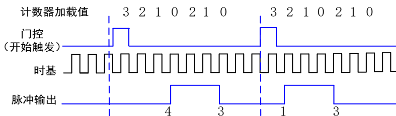
图 6-8-5 重触发器上具有初始延时的重触发单脉冲产生设置值为 False 触发和第一个触发边沿之间的最小时间是时基的两个嘀嗒
