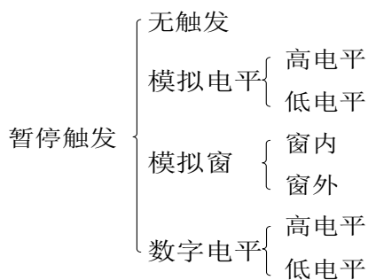
图 8-2-7 暂停触发分类
