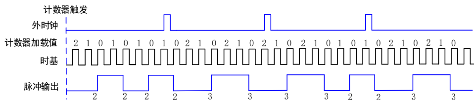
图 6-8-8 有限缓冲外时钟脉冲序列生成
