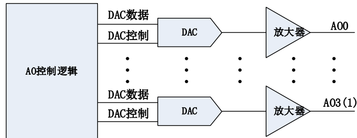
图 5-1-1 AO 功能框图
