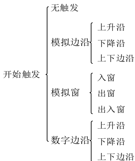
图 8-2-1 开始触发分类
