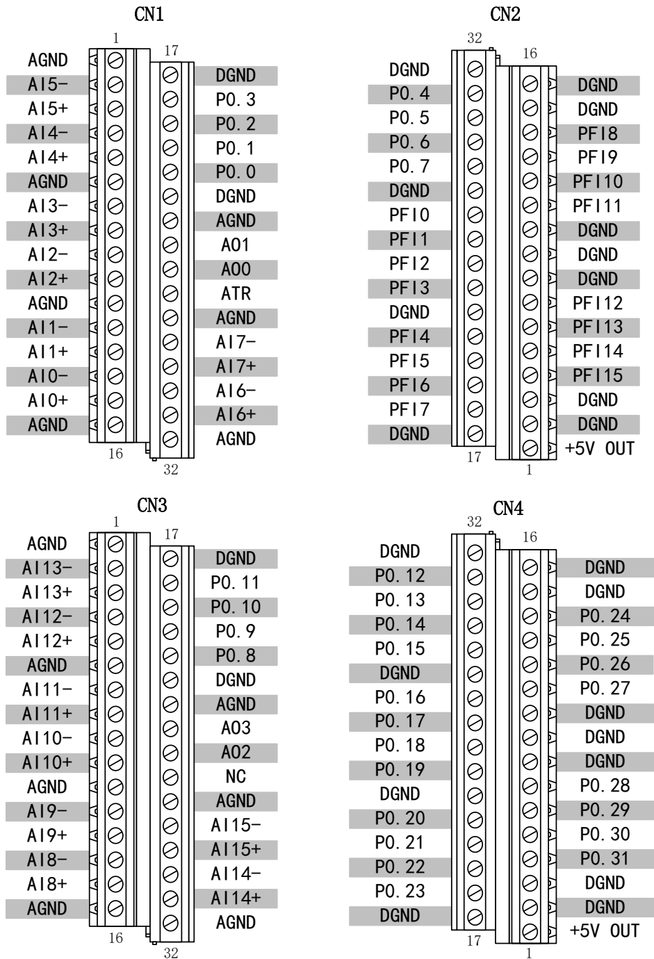
图 3-3-1 接线板管脚定义
