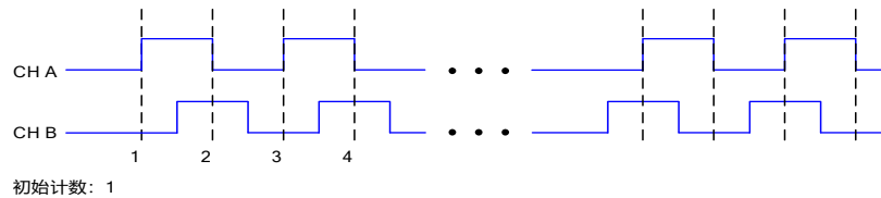
图 6-7-2 X2 编码
