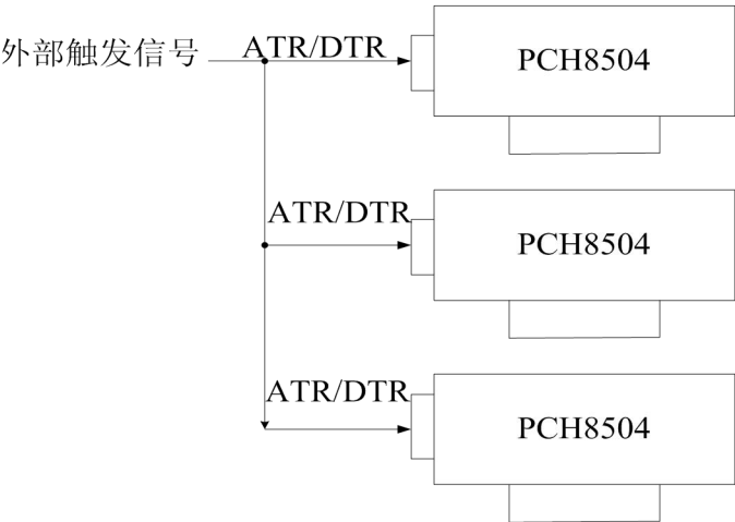
外触发同步采集的连接方法
