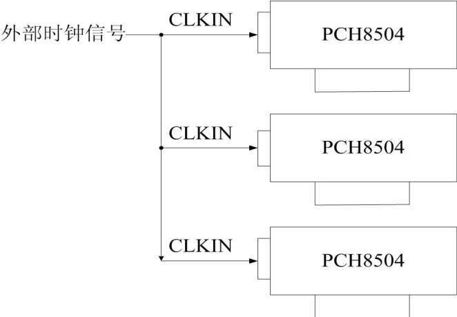
外时钟同步采集的连接方法
