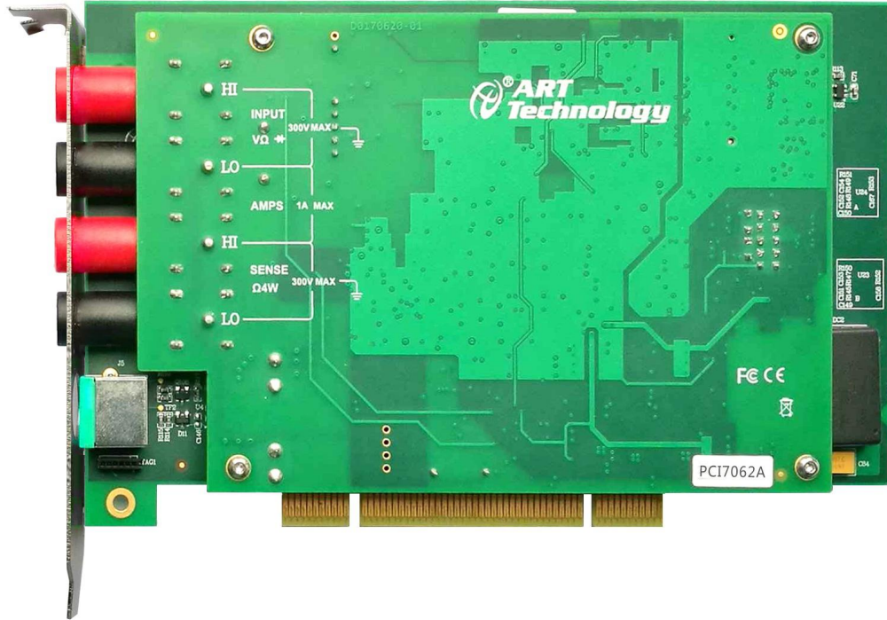
图 2-1-1 板卡外形图
