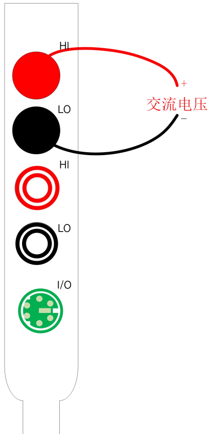
图 3-1-1 测量交流电压接线方式
