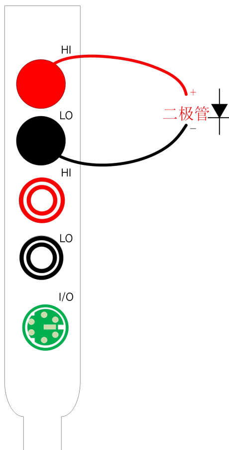
图 3-4 二极管测量接线方式
