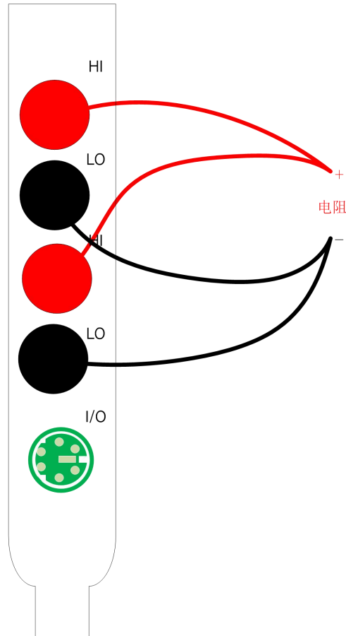
图 3-7 4W 电阻测量接线方式
