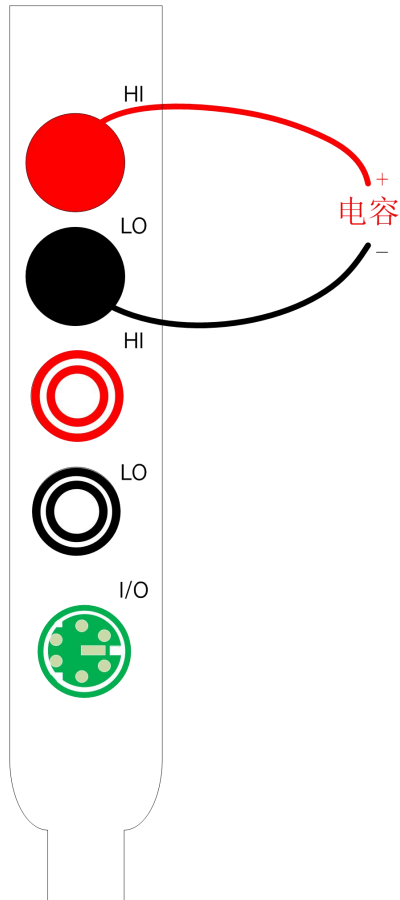
图 3-5 测量电容接线方式
