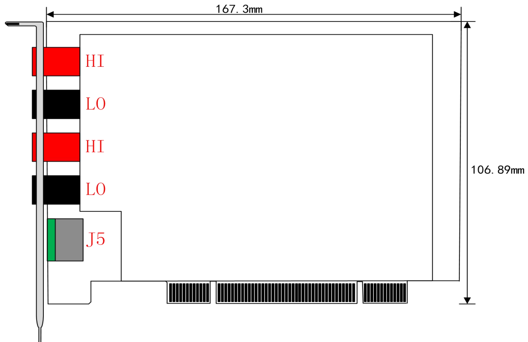
图 2-2-1 板卡尺寸图
