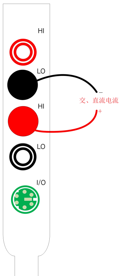
图 3-8 测量交、直流电流接线方式
