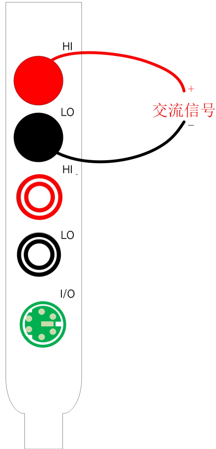
图 3-3 测量逻辑频率接线方式
