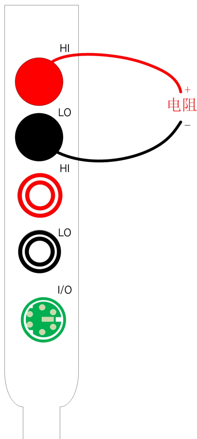
图 3-6 2W 电阻测量接线方式
