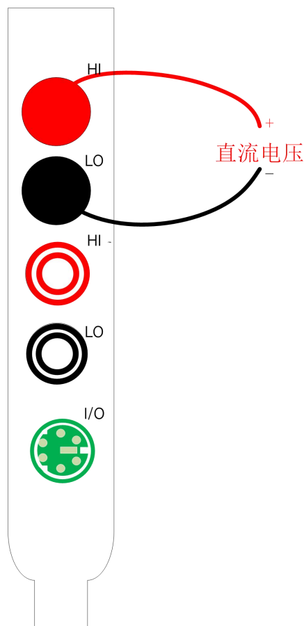
图 3-2 测量直流电压接线方式
