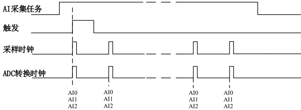
图4-6-3 连续采样
