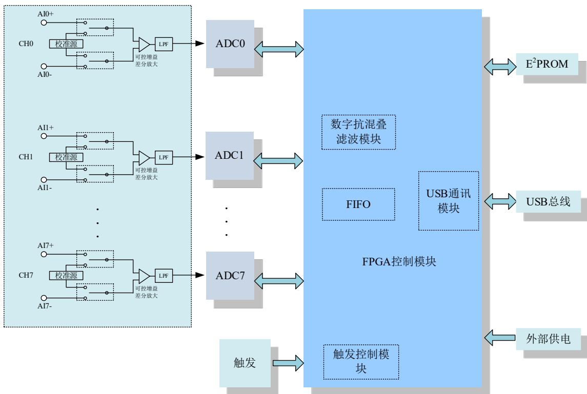
图 2-2-1 USB8860 系统框图
