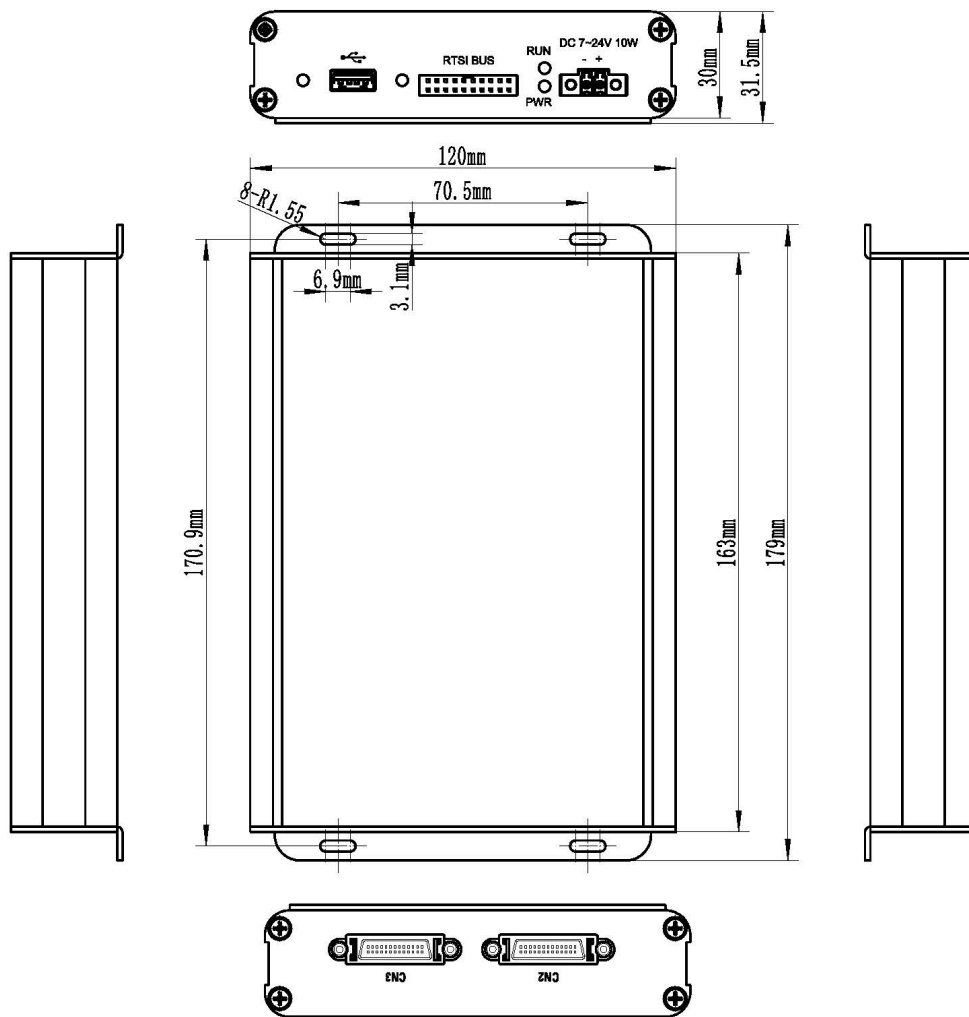
图 3-2-1 USB8860 外壳尺寸图
