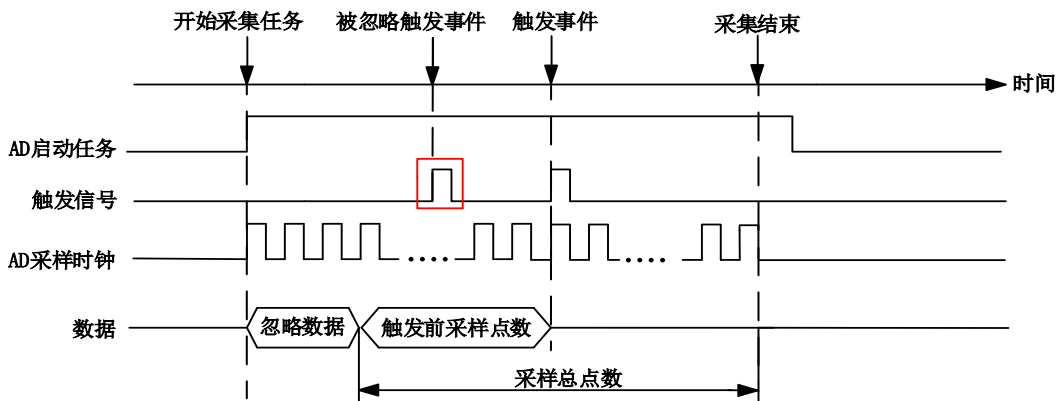
图 4-7-8 参考触发
