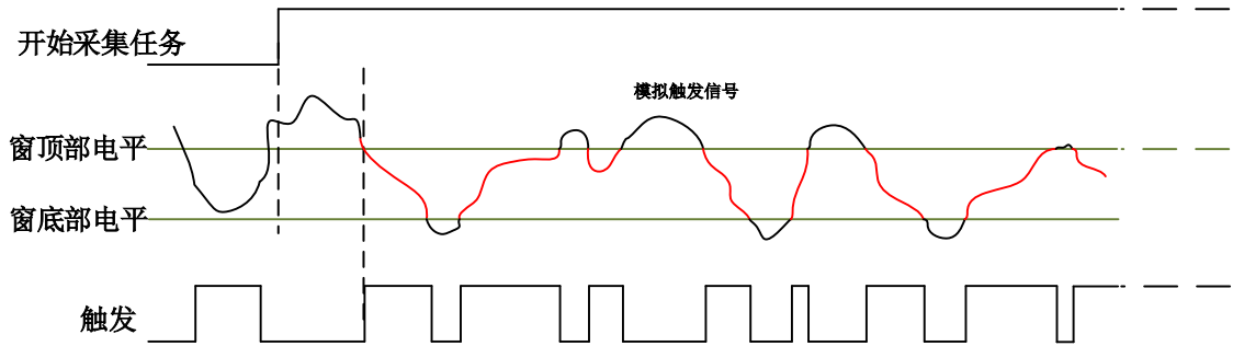
图4-8-9 模拟窗触发--入窗
