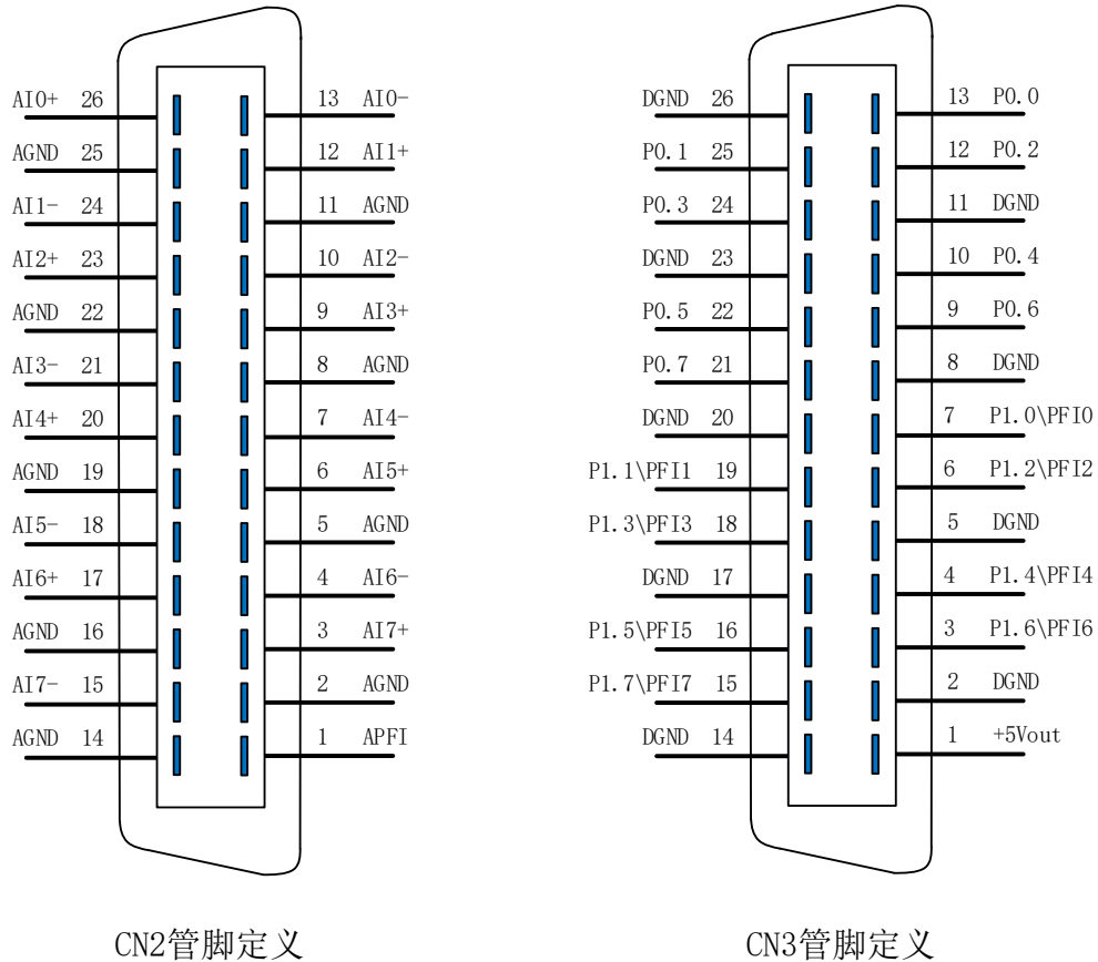
图 3-3-1 USB8860 接口定义
