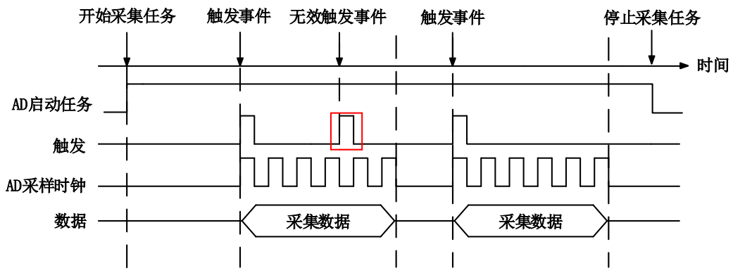
图 4-7-6 重触发
