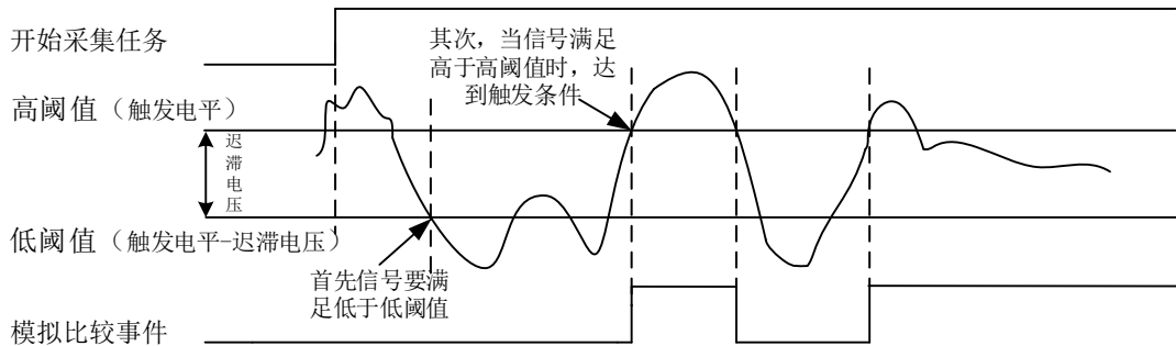
图4-8-7 模拟边沿迟滞触发—上升沿
