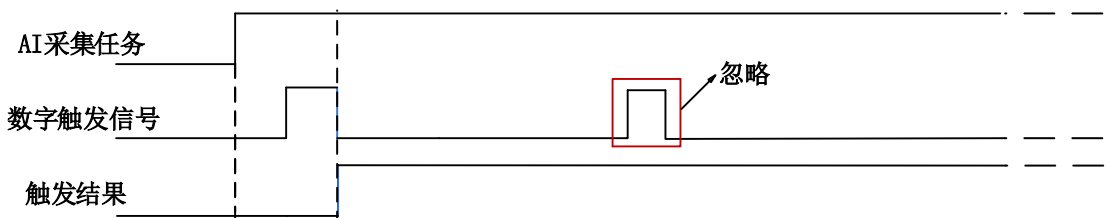
图4-8-11 数字边沿触发--下降沿触发
