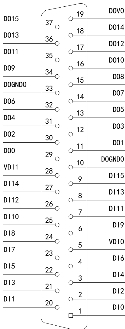
图 3-3-1 PCI2312B 接口定义
