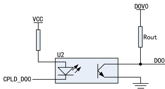
图 4-3-1 输出原理
