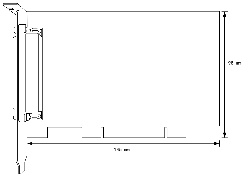
图 3-1-1 PCI2312B 尺寸图
