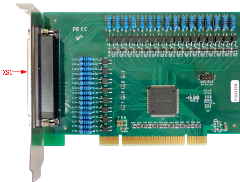
图 3-2-1 PCI2312B 元件布局图
