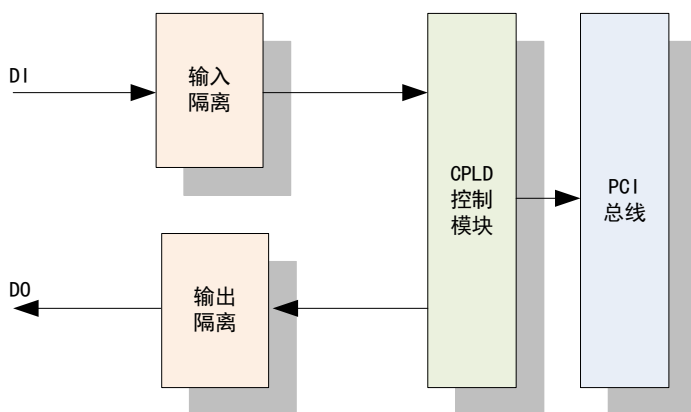
图 2-2-1 PCI2312B 系统框图
