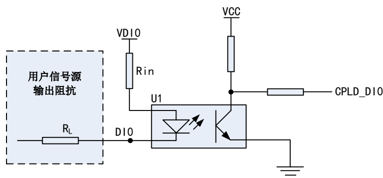
图 4-1-1 输入原理
