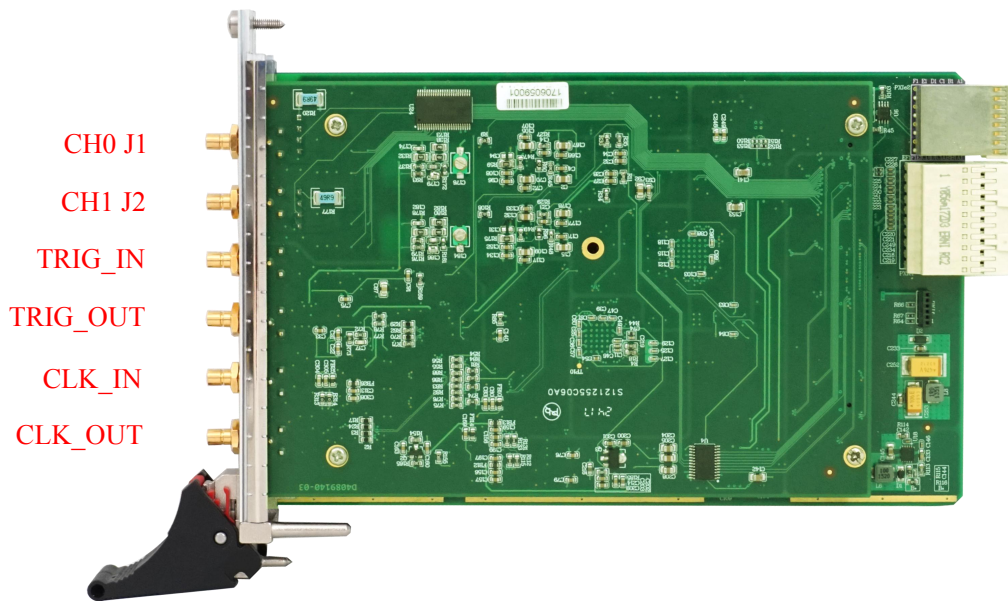
图 3-3-1 PXIe8914/8912 产品外观图
