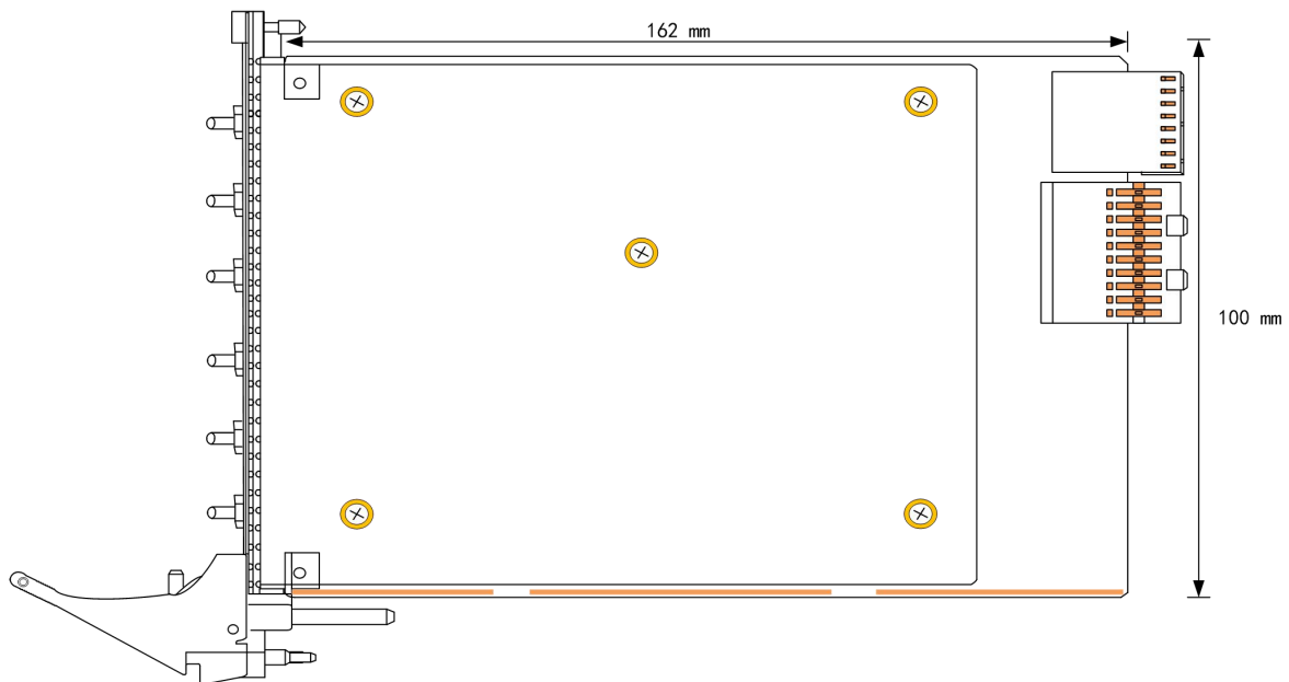
图 3-2-1 PXIe8914\8912 板卡尺寸图
