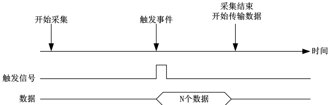
图 4-9-2-3 后触发
