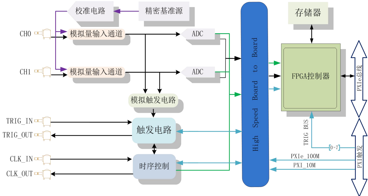
图 3-1-1 PXIe8914\8912 系统框图
