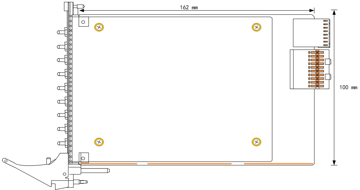
图 3-2-1 PXIe8582\8584\8586 板卡尺寸图
