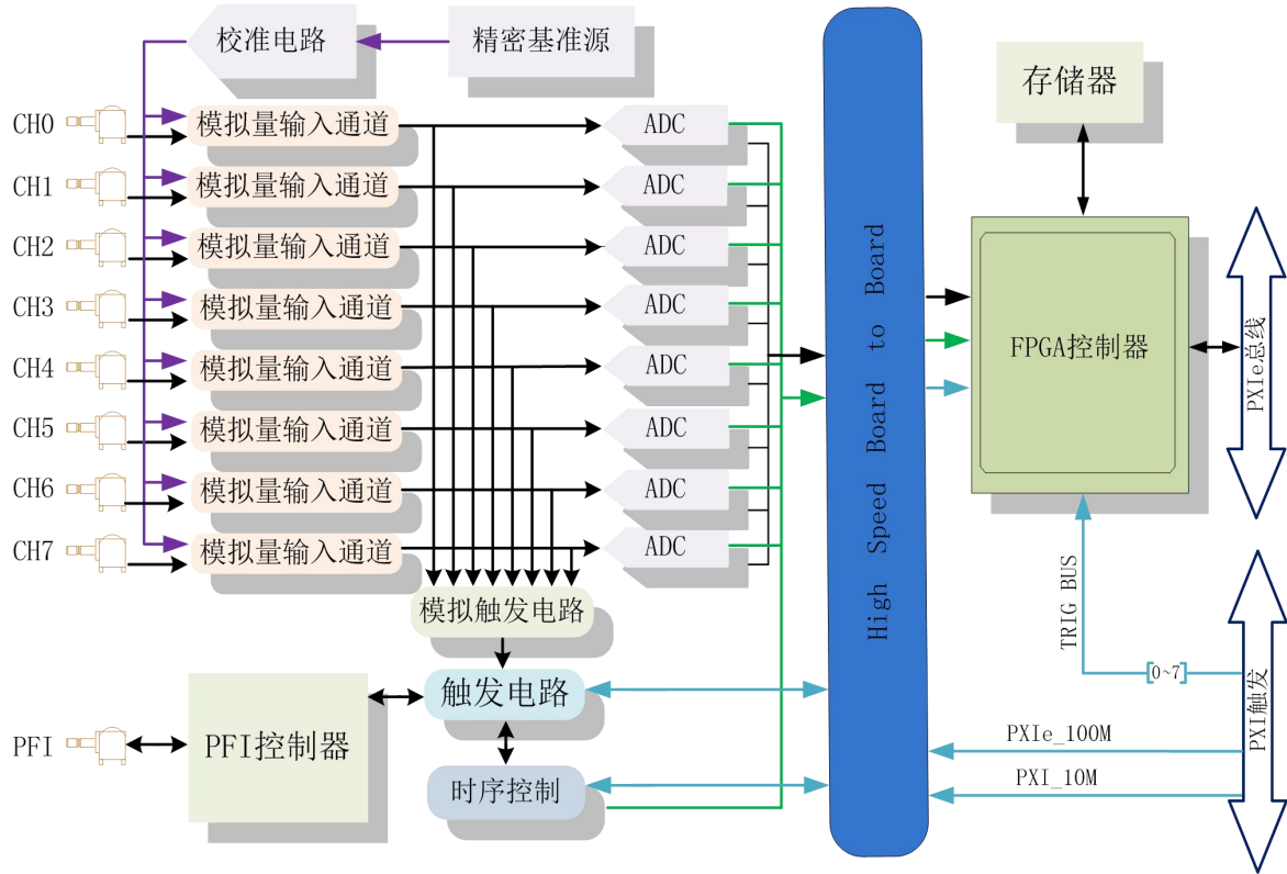
图 3-1-1 PXIe8582\8584\8586 系统框图
