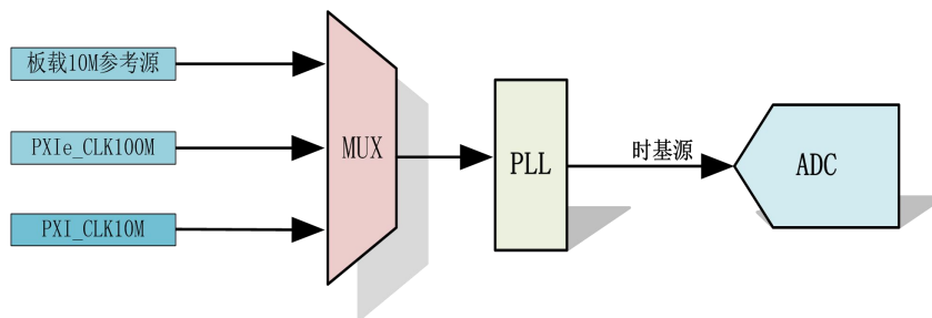
图 4-7-1 时基源框图
