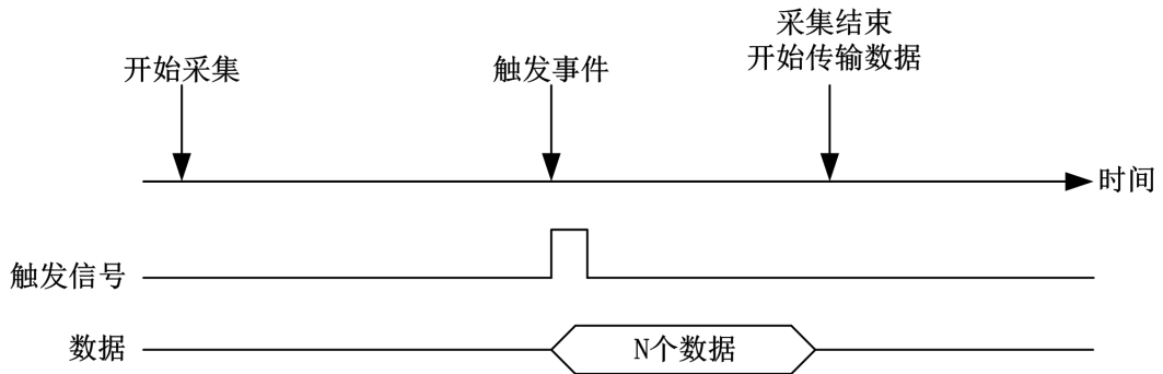
图 4-9-2-3 后触发
