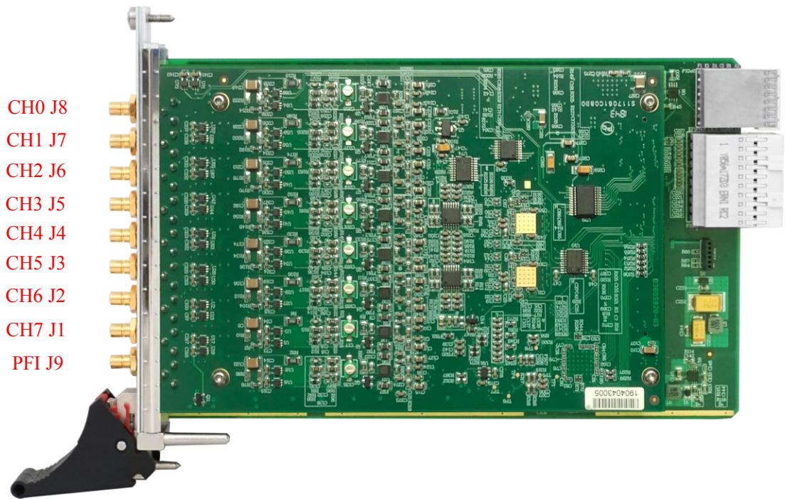
图 3-3-1 PXIe8582\8584\8586 产品外观图
