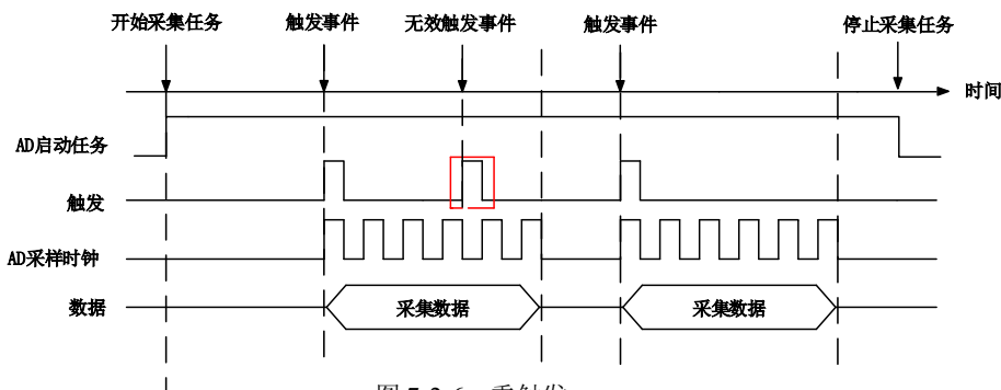
图 7-2-6 重触发
