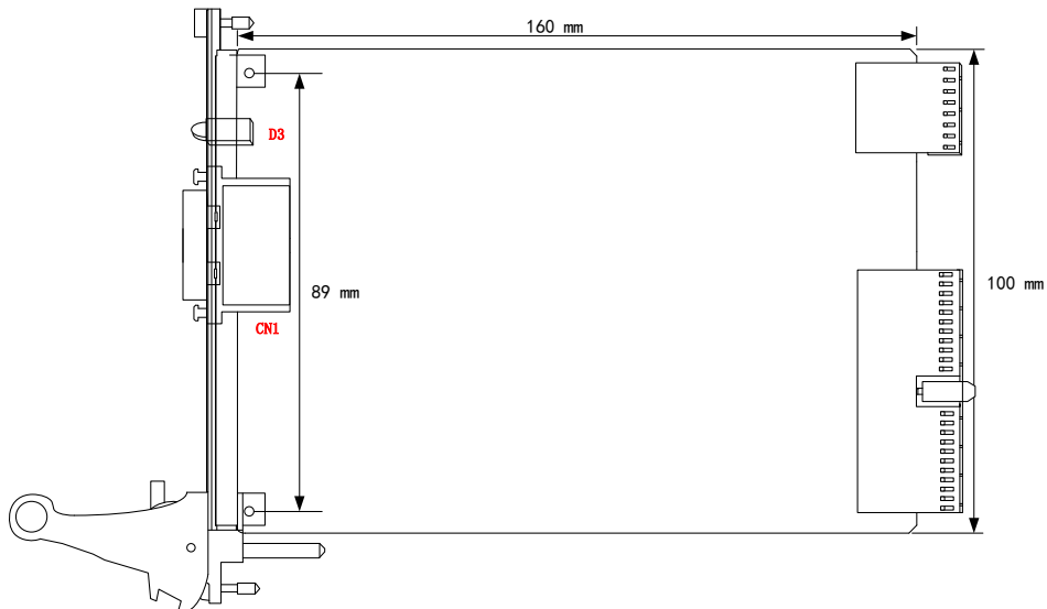
图 3-2-1 PXI9009\A/B 板卡尺寸图
