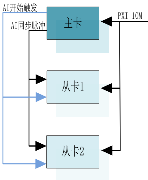
图 4-9-1 主从卡级联
