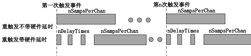
图 7-2-5 AI 重触发
